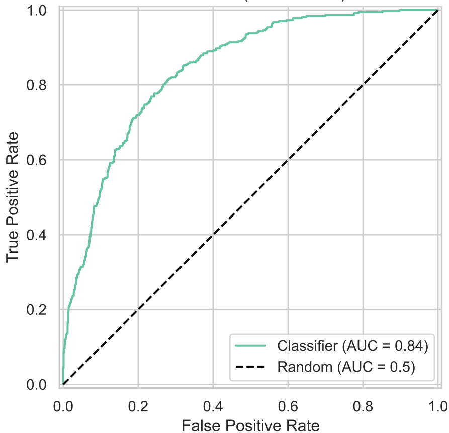
ROC Curve (AUC = 0.842)
