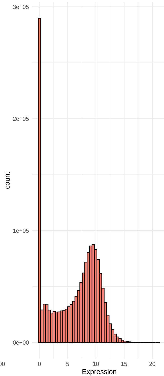
Distribución \log_2(\text{TPM} + 1)
