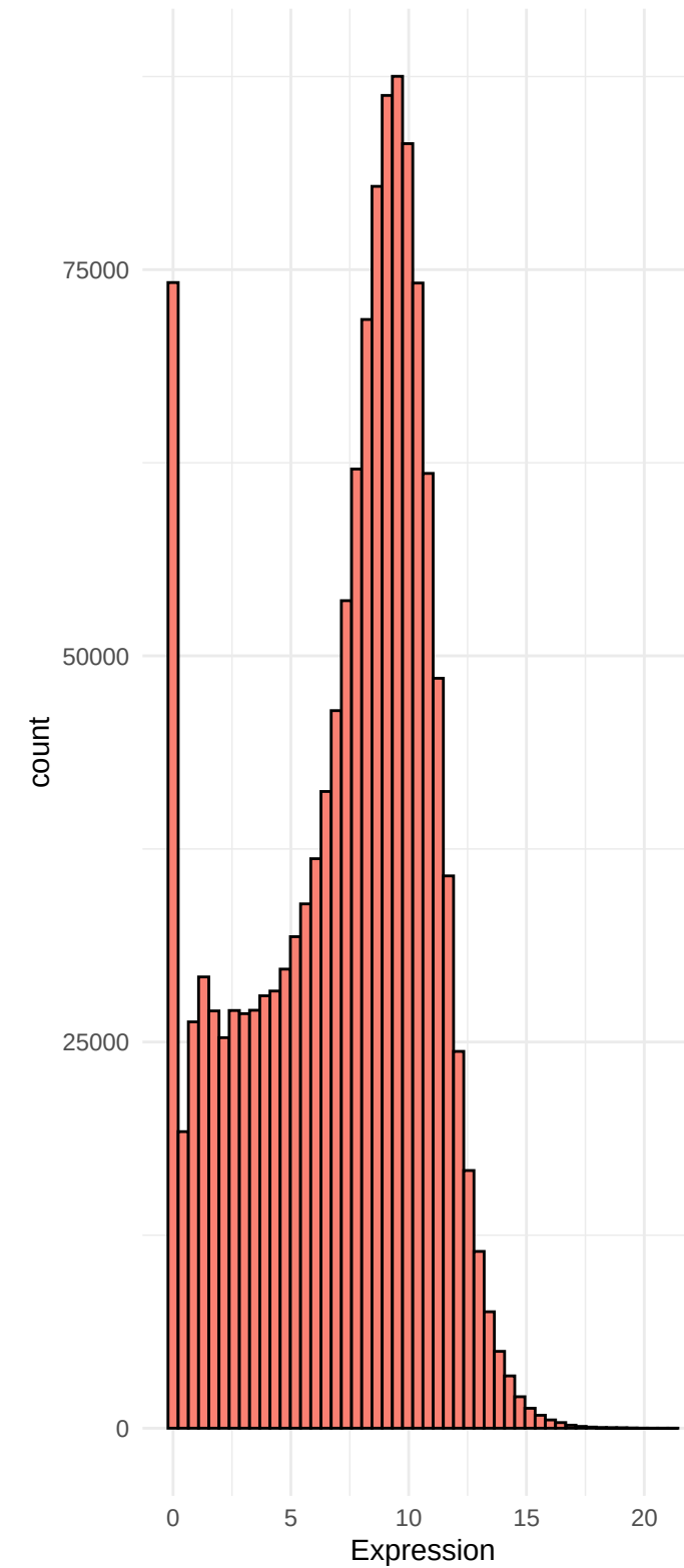
Distribución \log_2(\text{TPM} + 1) Filtered
