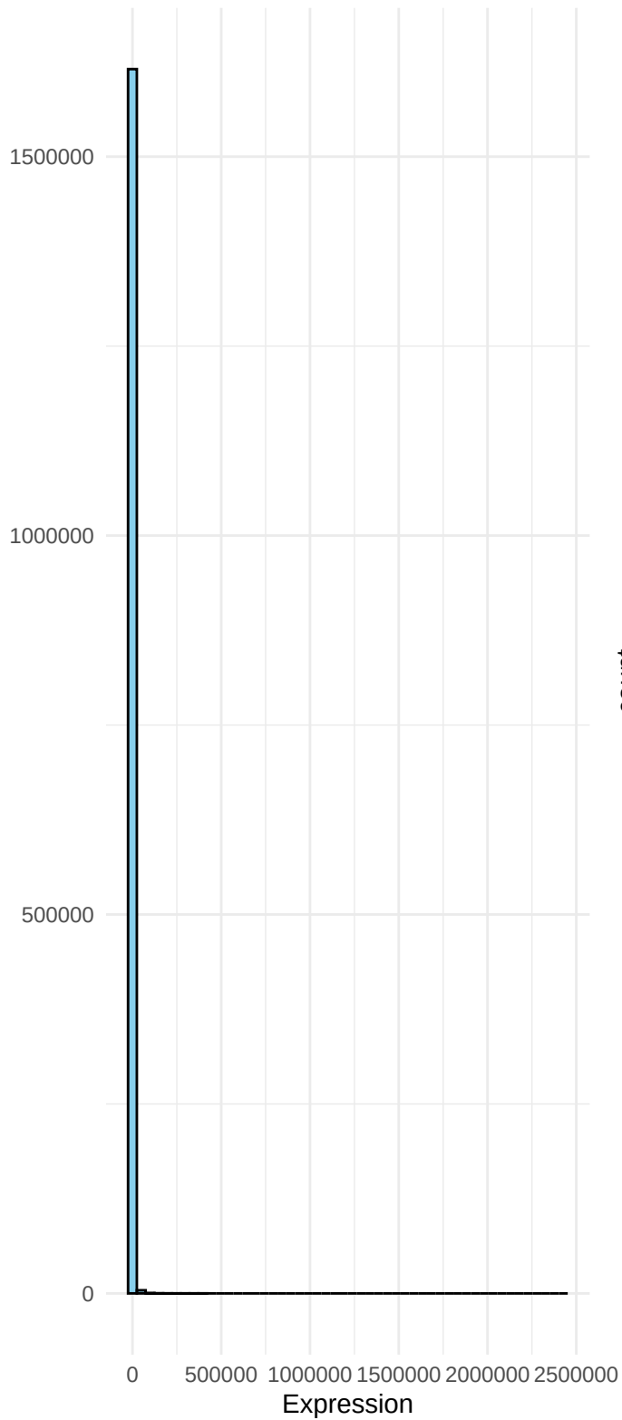
Distribución TPM
