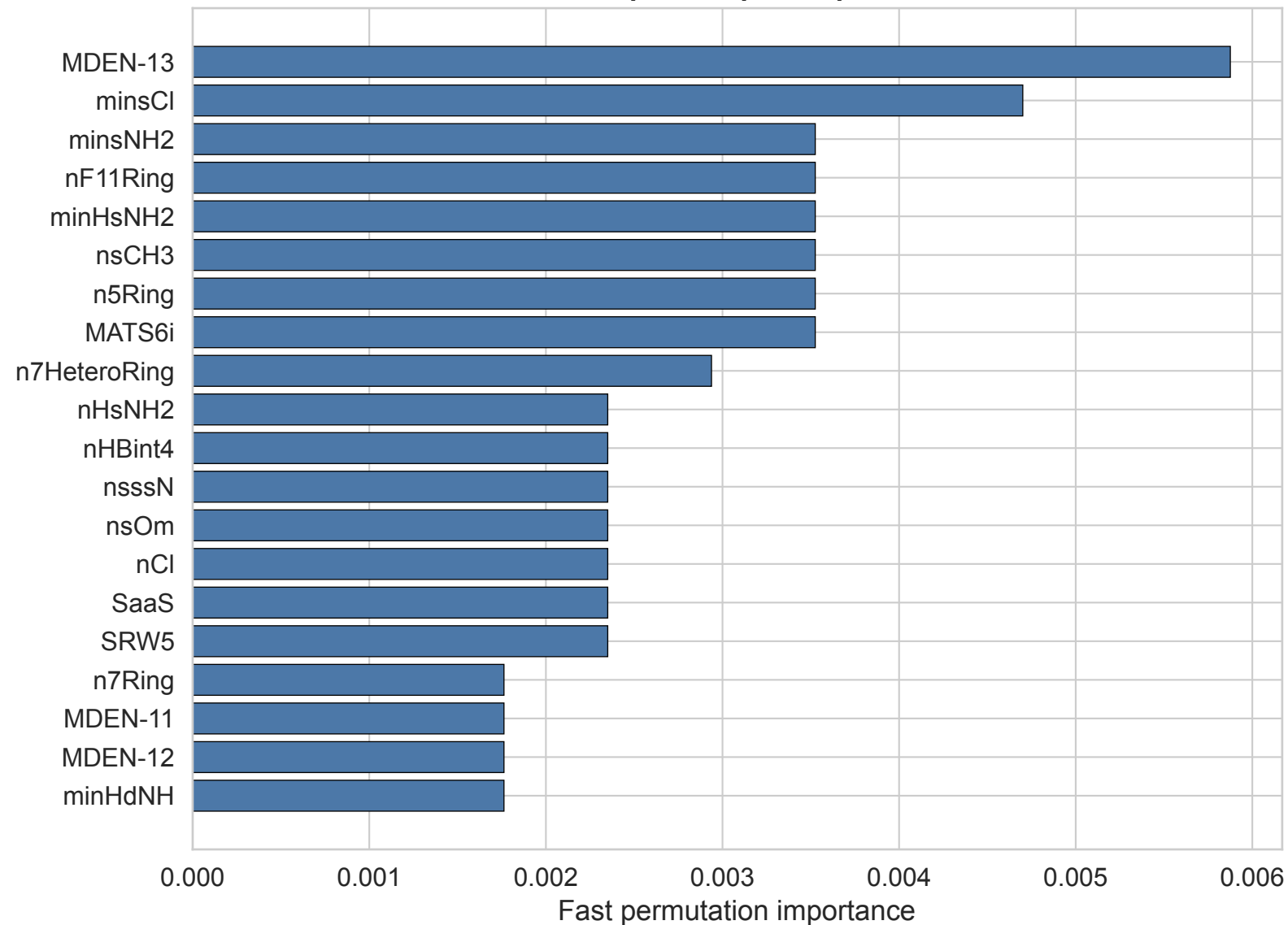
KNN: Top Descriptor Importance
