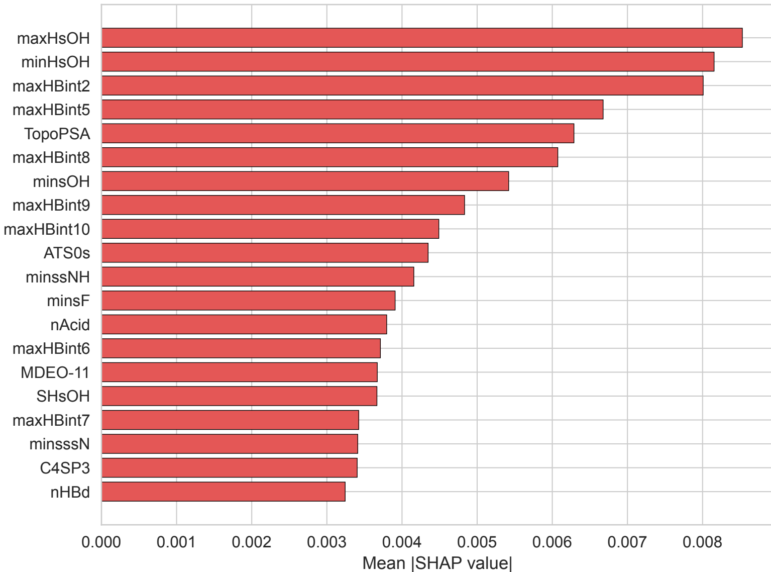
ET: Mean Absolute SHAP Values
