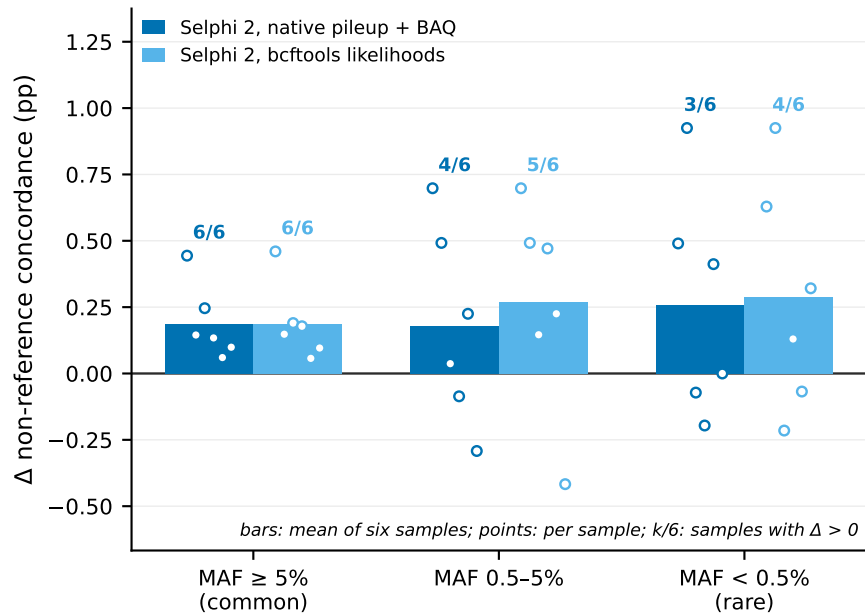
(d) Selphi 2 - GLIMPSE2 by reference-panel MAF
