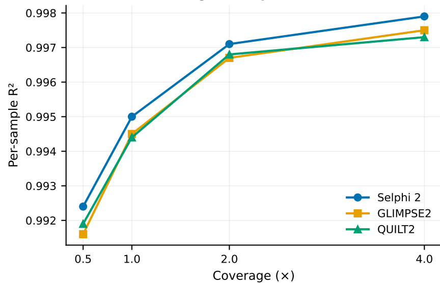
(d) IcWGS coverage sweep (GIAB)
