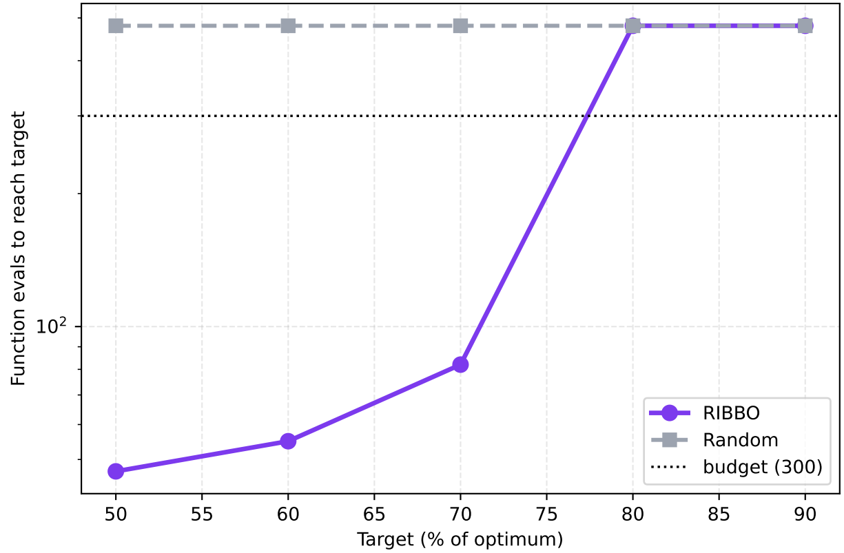
EE D=10 (3BA, 300)
