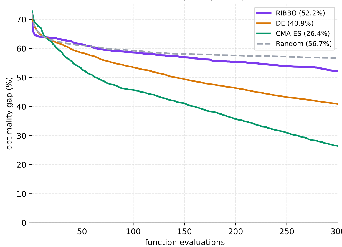
IFC SE D=10 (3BA) (200 ch)
