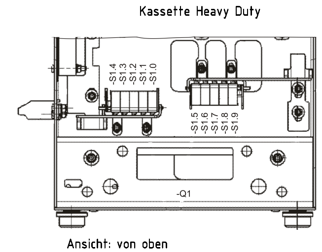
Betriebsmittel-Kennzeichnung / Item designation:
