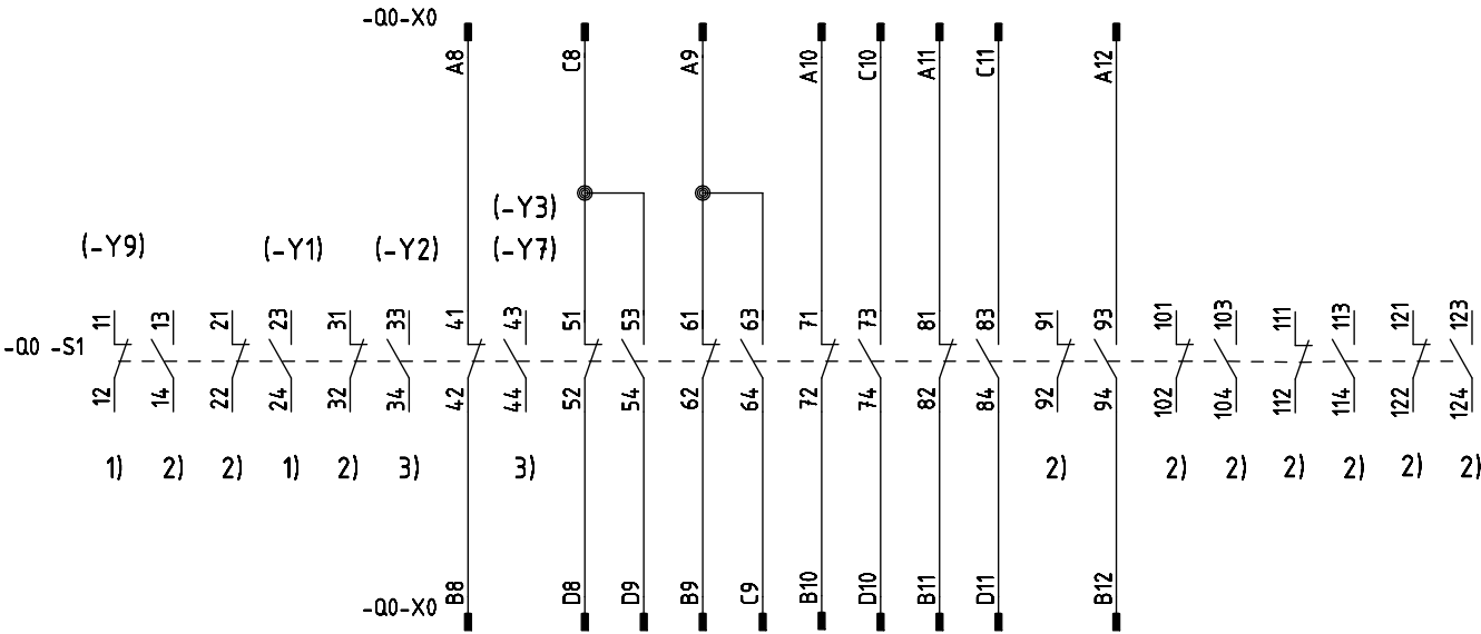
S_A7E_449_41063_004 Zusatz / Order code: W63 (nur 3AE5)
