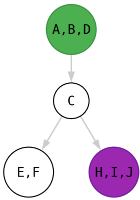
Граф Герца
