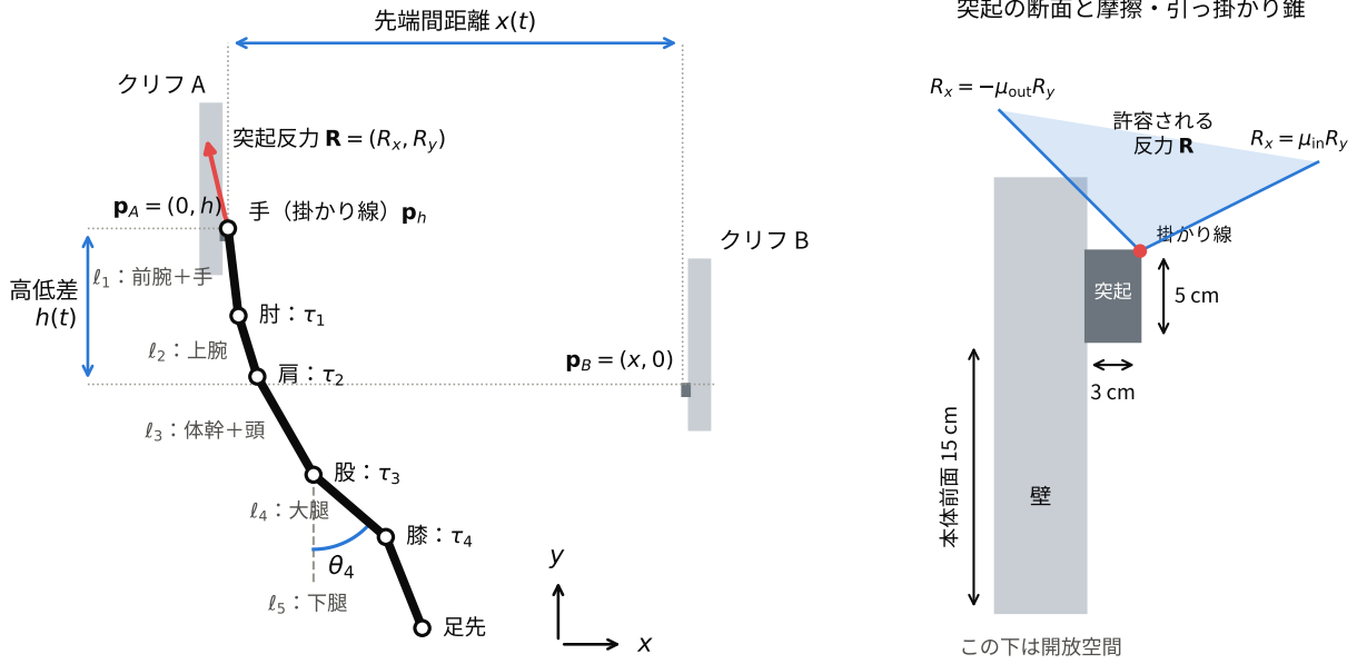
図 3 平面 5 リンク人体モデルと記号 (左), 突起の断面と反力の許容範囲 (右). 各リンクの角度 \theta_i は鉛直下向きから測る (図は大腿の \theta_4 を例示). 関節トルク \tau_1, \dots, \tau_4 は肘・肩・股・膝に働く. 手は突起の先端上縁の掛かり線 p_h に掛かり, 突起から反力 \mathbf{R} を受ける. 右図の青い領域は, 突起が手に及ぼせる反力の範囲 (摩擦・引っ掛かり錐) で, 壁から離れる向きには \mu_{\text{out}} R_y , 壁へ向かう向きには \mu_{\text{in}} R_y までの水平力を支えられる.
