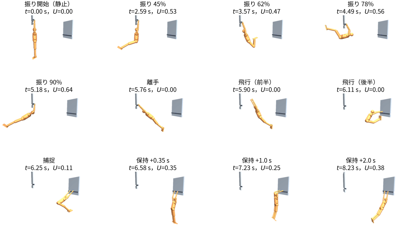
図 11 環境での実行例 ( T = 18 \text{ s} , m = 66 \text{ kg} , \phi_\ell = 0.25 の参照解の再生; 制御周期 2 ms, 共通の着地反射). t は振り開始からの時間, U はその瞬間の把持利用率. 2 s の保持まで成功した試行で, 最大の把持利用率は 1.51 であった.
