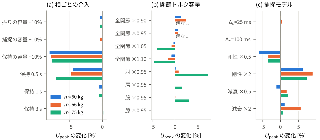
図 9 制約や能力を変えて解き直したときの必要把持容量の変化 (実験 9; T = 18 \text{ s} , \phi_\ell = 0.25 ). (a) 一つの相だけ把持容量の上限を 10% 緩めた場合と, 保持時間を変えた場合. (b) 関節トルク容量の上限を変えた場合. (c) 捕捉モデルを変えた場合 ( \Delta_c は剛体衝突モデル, 剛性と減衰は順応捕捉モデルで, それぞれのモデルの基準解に対する変化).
