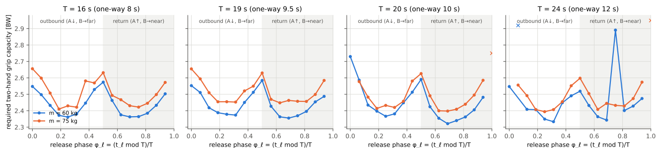
図 1 離手位相 \phi_l = (t_l \bmod T)/T と必要両手持持容量 (代表条件). 灰色は復路 ( \phi_l \geq 0.5 , A 上昇・B 接近). × は収束解が得られなかった条件 (いずれも装置折り返し点 \phi_l = 0 近傍).
