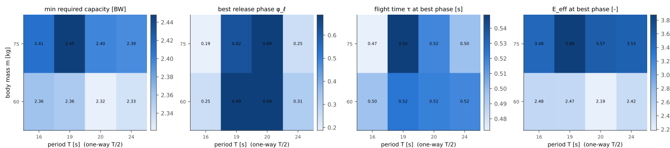
図 2 T \times m マップ (位相について最小化). 左から必要容量 [BW], 最良離手位相, 滞空時間, 努力指標.
