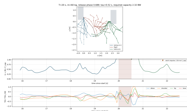
図 3 代表解 ( T = 20 s, m = 60 kg, 最良位相) のスティック図と把持利用率 U(t) . 青: A での振り, 赤: 飛行, 緑: B での保持. ▼ は捕捉負荷.
