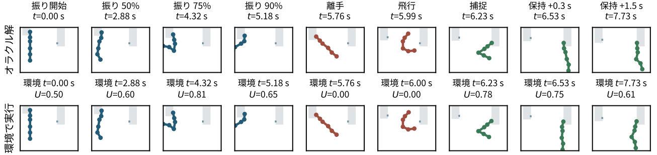
図 4 シミュレーションのスナップショット ( T = 18 \text{ s} , m = 66 \text{ kg} , \phi_\ell = 0.25 ). 上: オラクル解 (振り・飛行・保持). 下: 同じ解を環境で実行したもの (2ms 実行系+着地反射; B を捕捉して 2s の保持に成功した例). U は保持利用率.
