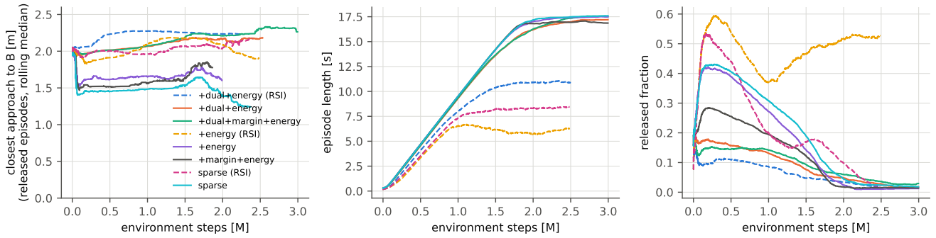
図5 PPOの学習曲線（移動平均，破線は参照状態初期化）：離手したエピソードの手先とB先端の最接近距離，エピソード長，離手率．最接近距離はどの条件でも1.3mを下回らず（オラクル解では2cm以内），学習は「期限まで静止」へ収束する．
