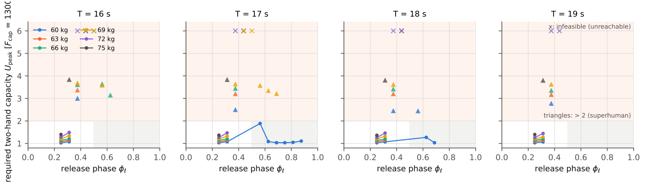
図 2 離手位相 \phi_\ell と必要両手持持容量（修正モデル，98 条件計算済み；グリッドは計算継続中）． \Delta は 2（両手 2600 N，超人的）を超える解， \times は実行不能（到達不足），灰色は復路．
