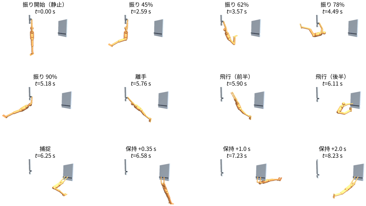
図 4 最適解の 3 次元連続図 ( T = 18\text{ s} , m = 66\text{ kg} , \phi_\ell = 0.25 ). t は振り開始からの時間. 各コマの装置はその時刻の位置にある (A は下降し, B は遠ざかる). 平面モデルは体の向きの反転を空中で自由に行えるとするので, 飛行の前半は A 向き, 後半は B 向きで描いた. 矢状面内の関節の位置はモデルの解そのものである.
