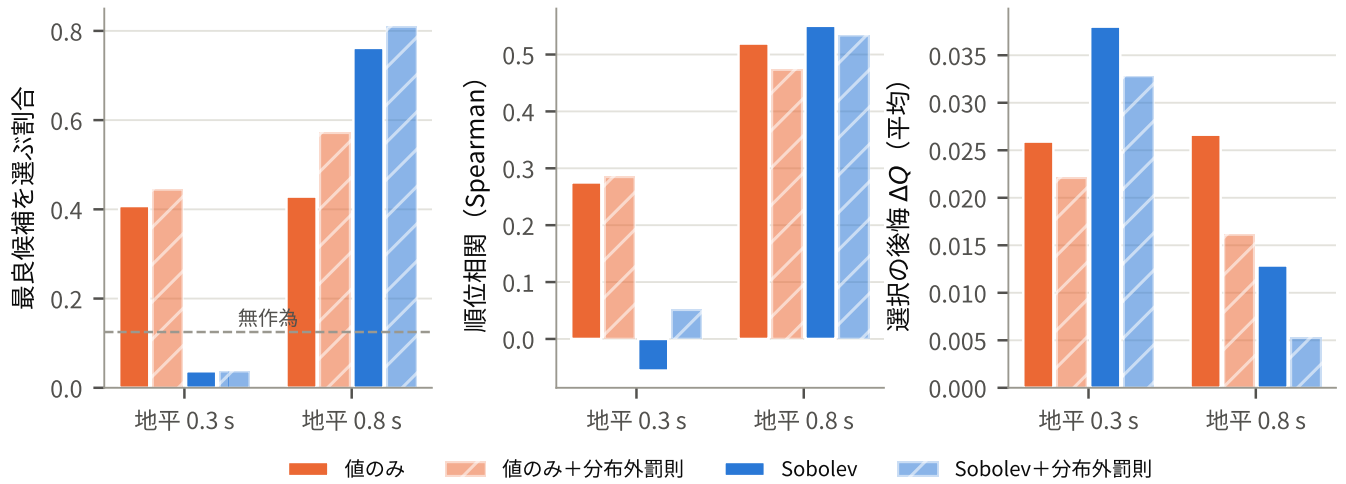
図 16 候補の順位付け (実験 5). 10 状態 × 8 候補 × 3 回の学習. 左: 最良の候補を選んだ割合 (破線は無作為に選んだ場合). 中: 場による順位とオラクルによる順位の間. 右: 選んだ候補と最良の候補の評価値の差. 斜線は分布外の罰則を加えた場合.
