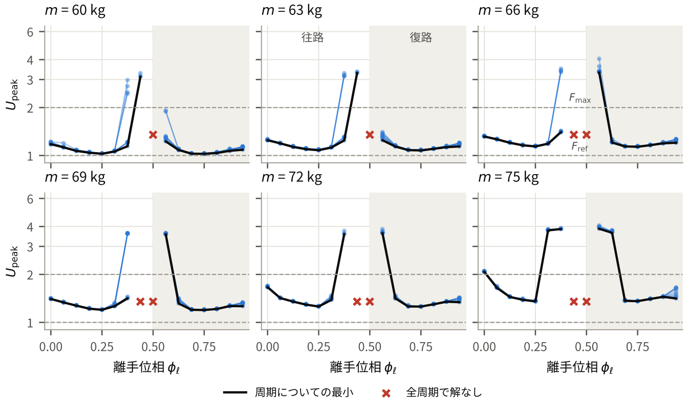
図 6 離手位相 \phi_l と必要把持容量 U_{\text{peak}} (体重ごと). 細い青線は 9 通りの装置周期のそれぞれ, 太い黒線は周期についての最小値. \times はどの周期でも解が得られなかった位相. 破線は F_{\text{ref}} ( U_{\text{peak}} = 1 ) と見出しの許容容量 F_{\text{max}} ( U_{\text{peak}} = 2 ). 灰色の背景は復路. 縦軸は対数.
