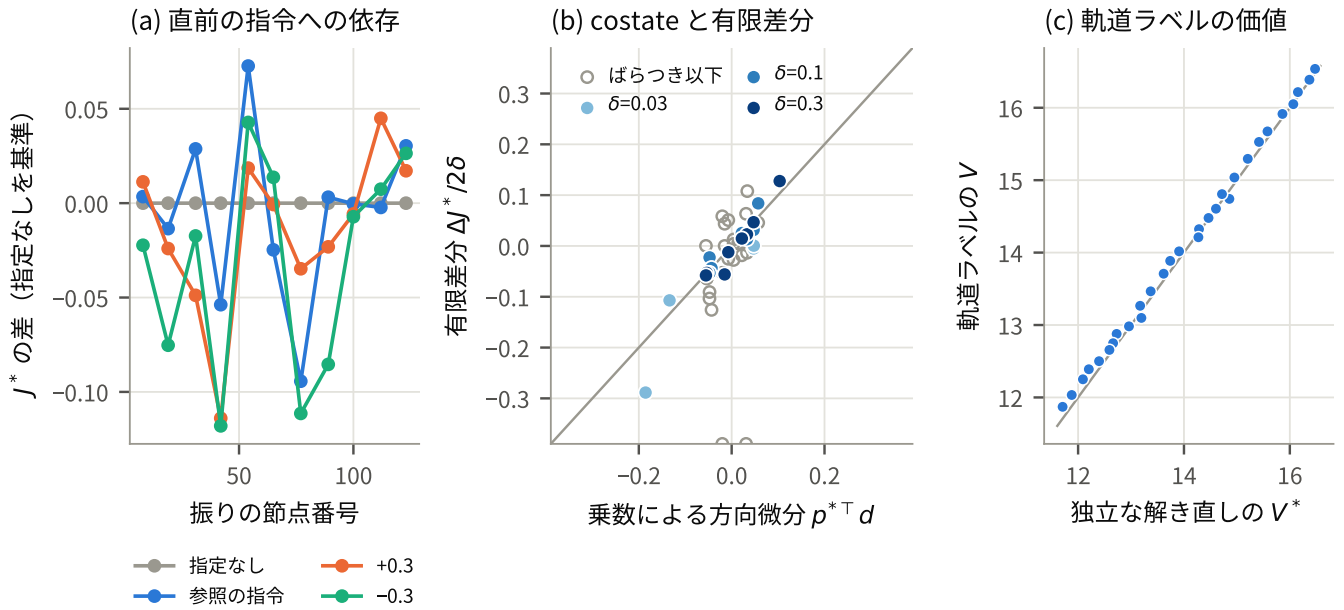
図 15 双対ラベルの検査（実験 4）．(a) 直前の指令を変えて解き直したときの J^* の差．(b) costate による方向微分（横軸）と，解き直しによる有限差分（縦軸）．刻み \delta \geq 0.03 の組を示す．色のついた点は costate による変化が解き直しのばらつきを上回った組，白抜きの点はばらつき以下の組（縦軸の範囲で切っている）．対角線に乗れば一致．(c) 軌道の節点から作った価値ラベルと，その状態から独立に解き直した価値．
