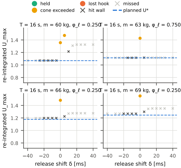
図 6 離手指令のずれ \delta に対する再積分結果 (代表 4 条件). 丸は掌が掛かった試行, \times は捕捉失敗. 破線は計画値 U^* .
