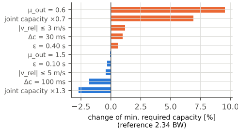
図 7 一因子感度: 位相について最小化した必要容量の基準値からの変化.
