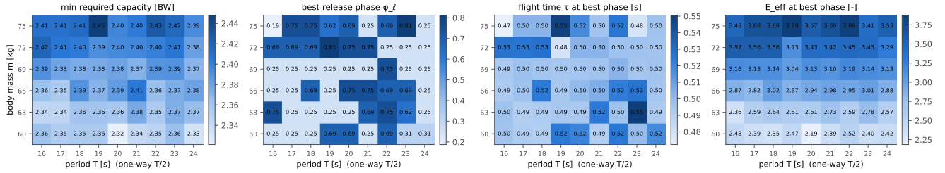
図3 T \times m マップ (位相について最小化). 左から必要容量 [BW], 最良離手位相, 滞空時間, 努力指標.
