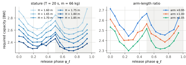
図4 体格掃引: 身長 H (左) と腕長比 (右) に対する必要容量の位相依存.
