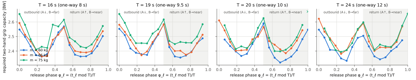
図2 離手位相 \phi_\ell = (t_\ell \bmod T)/T と必要両手持持容量 (代表条件). 灰色は復路. \times は収束解が得られなかった条件 (装置折り返し点 \phi_\ell = 0 近傍).
