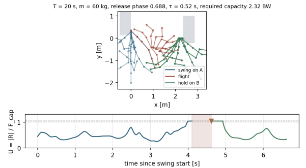
図5 代表解 ( T = 20 s, m = 60 kg, 最良位相) のスティック図と把持利用率 U(t) . 青: A での振り, 赤: 飛行, 緑: B での保持. \blacktriangledown は捕捉負荷, 破線は U_{\text{peak}} .
