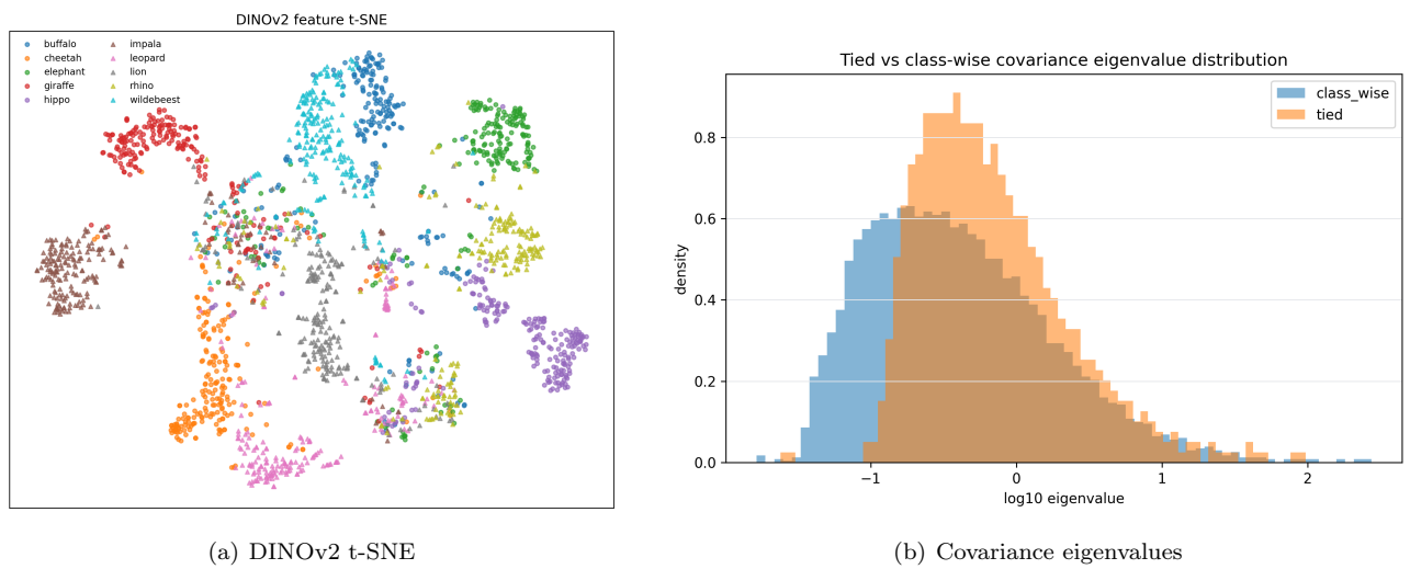
図 12: DINOv2 特徴空間の可視化と共分散固有値分布。
