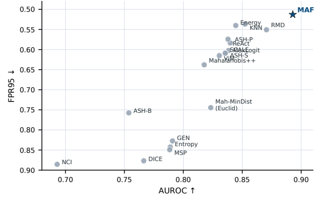
図 5: WILD_DATA における主要手法の AUROC と FPR95 の同時比較。MAF は高い AUROC と低い FPR95 を両立する。
