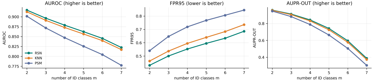
図2 ID クラス数 m = 2-7 に対する pooled AUROC, FPR95, AUPR-OUT. RSN は全 18 条件 (6 sizes \times 3 metrics) で KNN/PSM を上回る.
