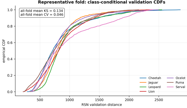
図 3 代表 fold のクラス別 validation 距離 CDF. 数値は全 1,476 fold の平均.
