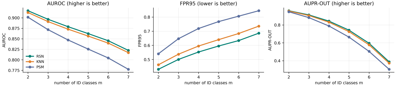
図2 ID クラス数 m = 2-7 に対する pooled AUROC, FPR95, AUPR-OUT. RSN は全 18 条件 (6 sizes \times 3 metrics) で比較手法を上回る.
