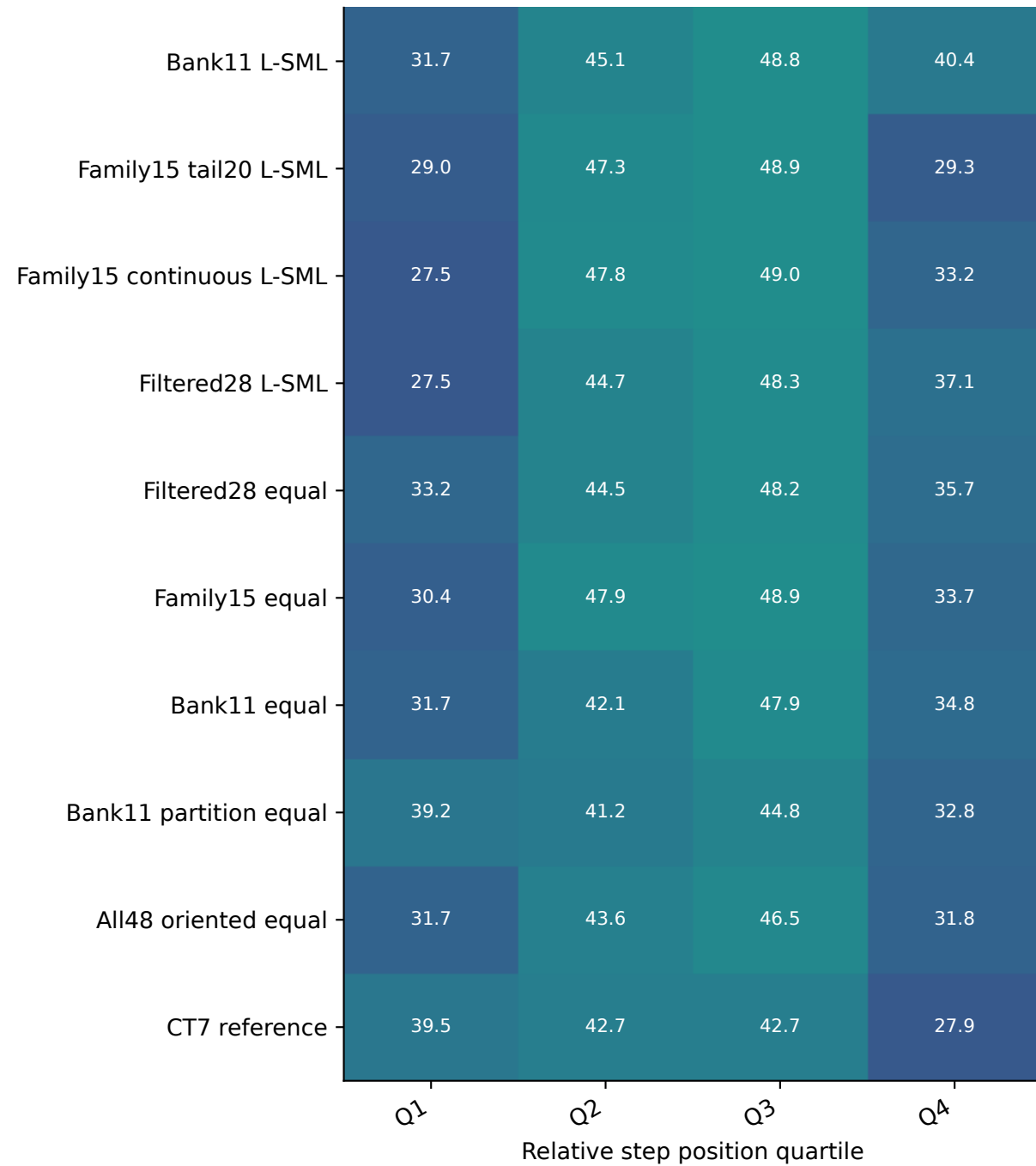
Hard2Verify / Qwen3-8B
