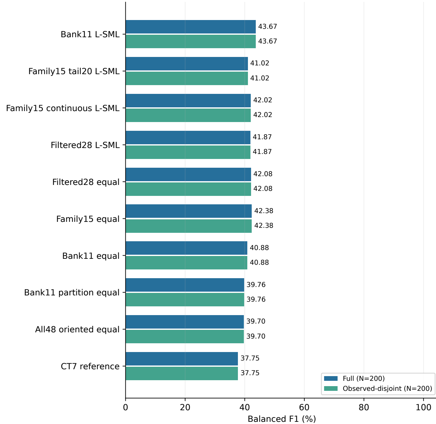
Hard2Verify / Qwen3-8B
