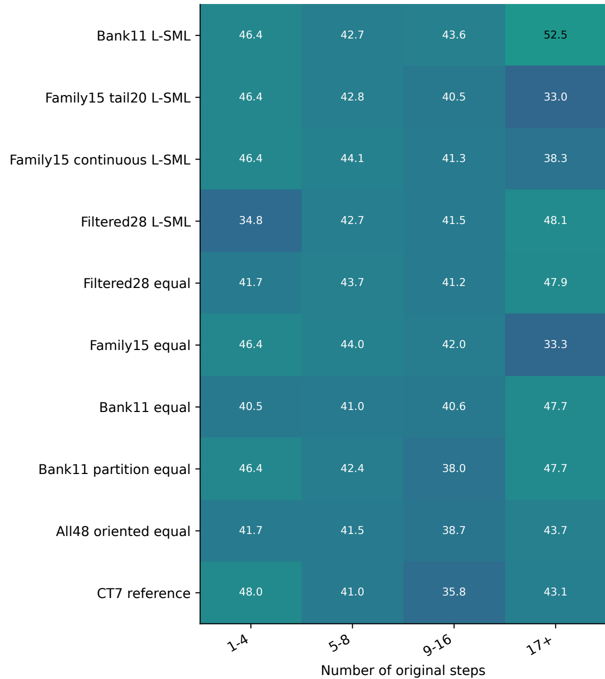
Hard2Verify / Qwen3-8B
