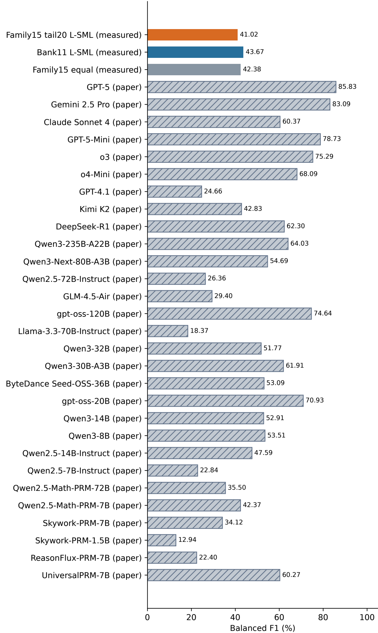
Hard2Verify / Qwen3-8B
