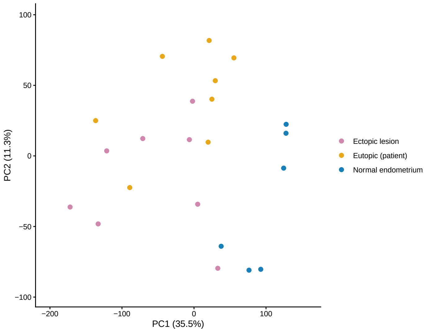
GSE25628 – PCA (n = 22)
