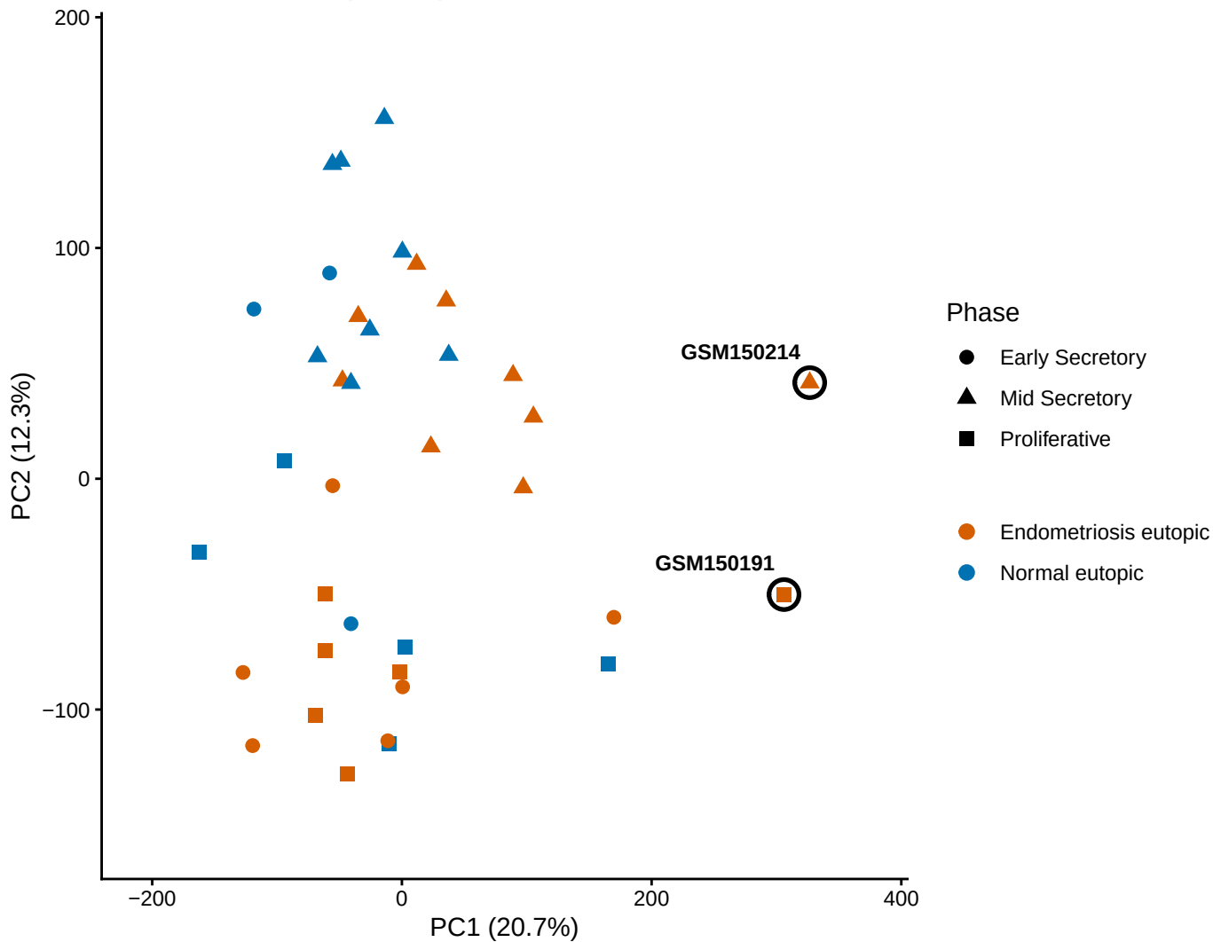
GSE6364 – PCA (n = 37)
