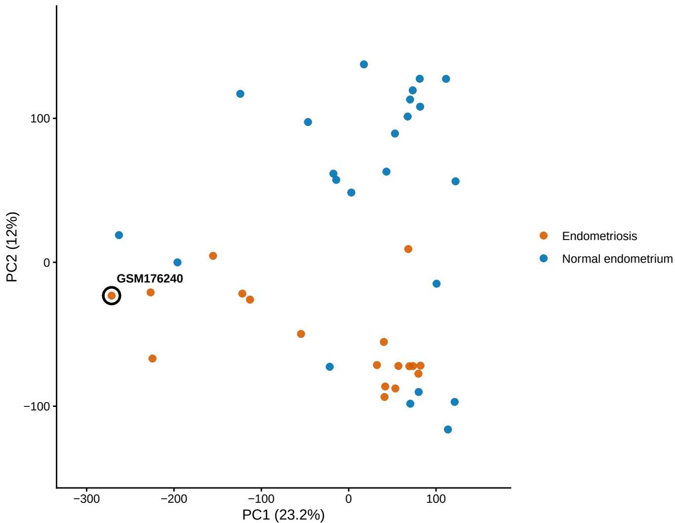
GSE7307 – PCA (n = 41)
