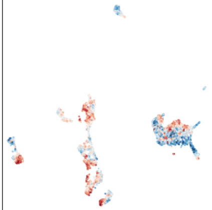
VAX1 (VAX1_MA0722.2)
