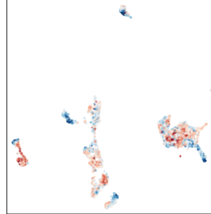
NACC2 (NACC2_MA2507.1)
