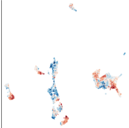
ZNF135 (ZNF135_MA1587.1)
