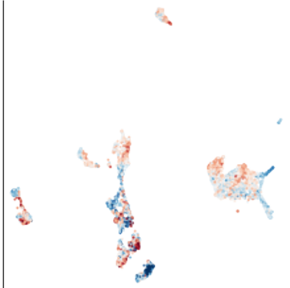
ZNF610 (ZNF610_MA1713.2)
