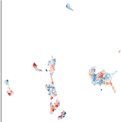
VSX1 (VSX1_MA0725.2)
