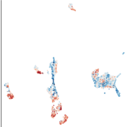
ZNF20 (ZNF20_MA2580.1)
