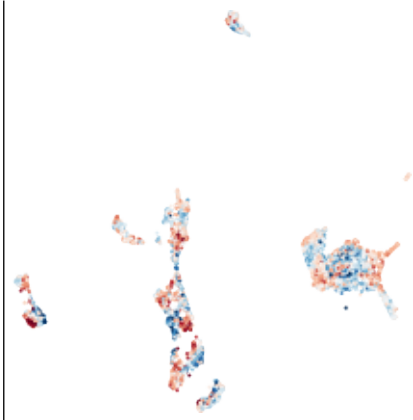
ZNF418 (ZNF418_MA1980.1)
