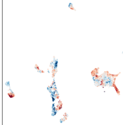
VSX2 (VSX2_MA0726.2)
