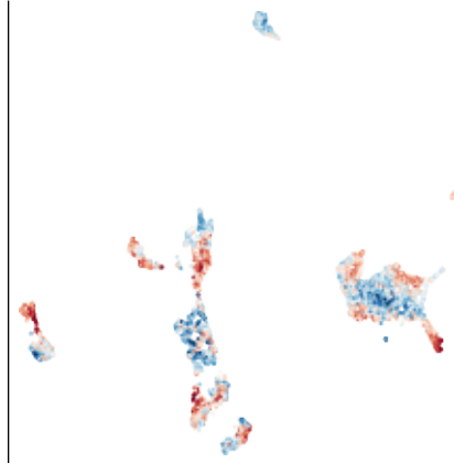
POU4F3 (POU4F3_MA0791.2)
