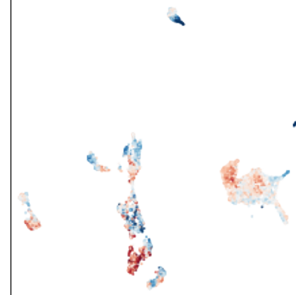
ZNF470 (ZNF470_MA2689.1)
