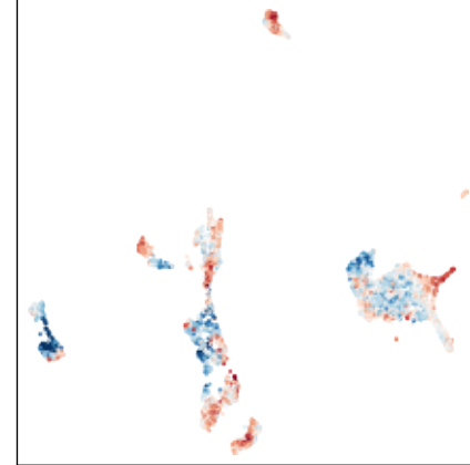
Gfi1B (Gfi1B_MA0483.2)
