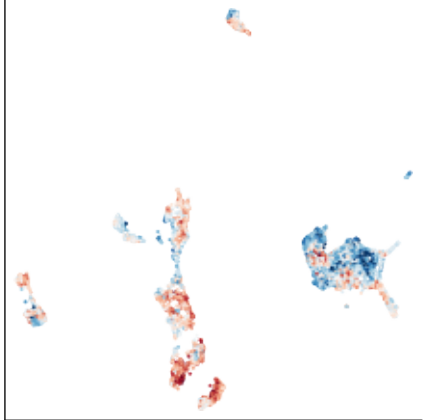
ZNF417 (ZNF417_MA1727.2)
