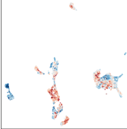
ZNF286B (ZNF286B_MA2551.1)
