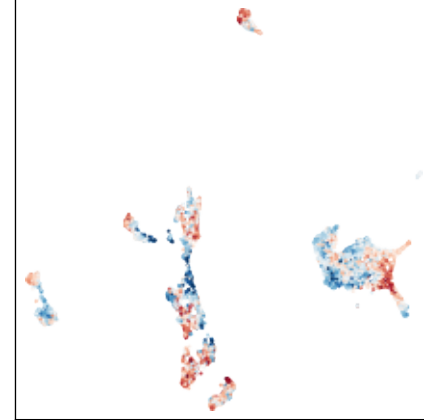
GLIS1 (GLIS1_MA0735.2)
