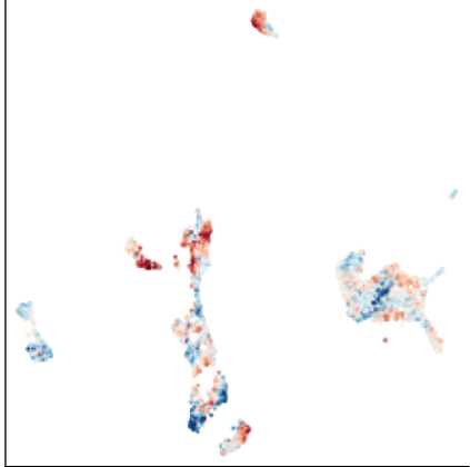
PAX2 (PAX2_MA0067.3)
