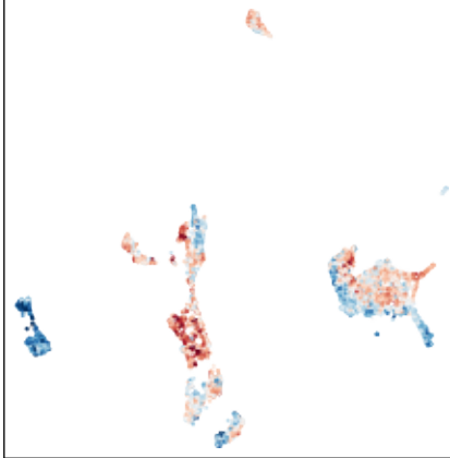
ZNF76 (ZNF76_MA1716.2)
