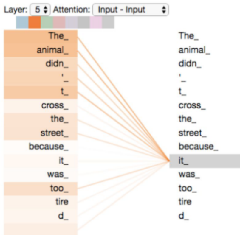
Figure 19: Self-attention позволяет токeну учитывать другие релевантные токены той же последовательности.
