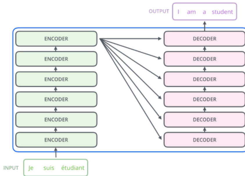
Figure 17: Transformer состоит из стека encoder-блоков и decoder-блоков.
