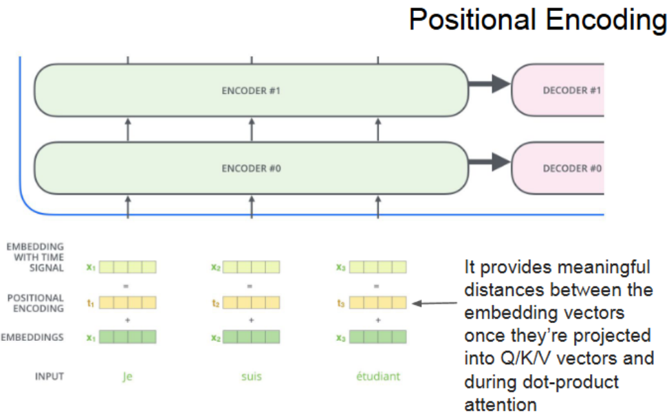
Figure 25: Positional encoding добавляет информацию о позиции токена к его embedding.
