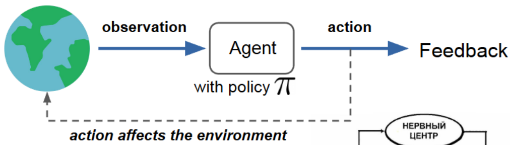
Figure 38: Основной цикл Reinforcement Learning: агент наблюдает состояние, выбирает действие и получает feedback от среды.
