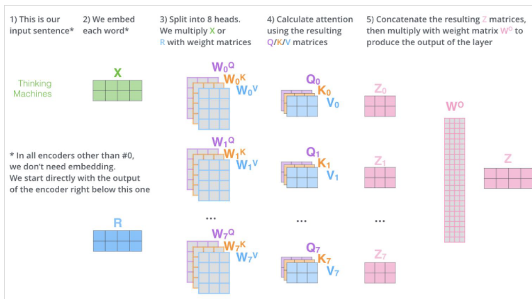
Figure 24: Multi-head attention: несколько attention-голов работают параллельно, затем их выходы объединяются.
