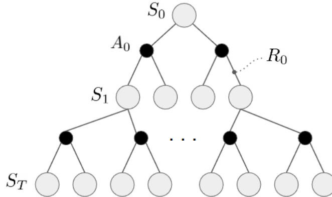
Figure 47: Backup tree показывает все возможные будущие траектории, но полный перебор обычно невозможен.
