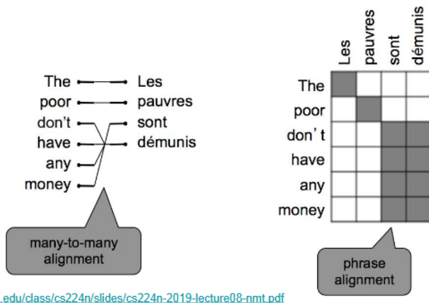
Figure 10: Пример many-to-many alignment: соответствие между фразами, а не отдельными словами.
