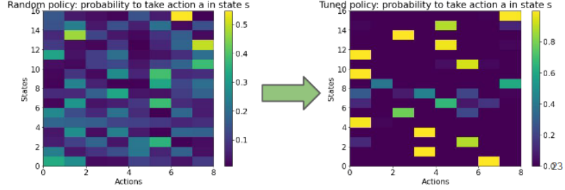
Figure 40: Cross-Entropy Method в табличном случае: policy matrix обновляется по elite sessions.
