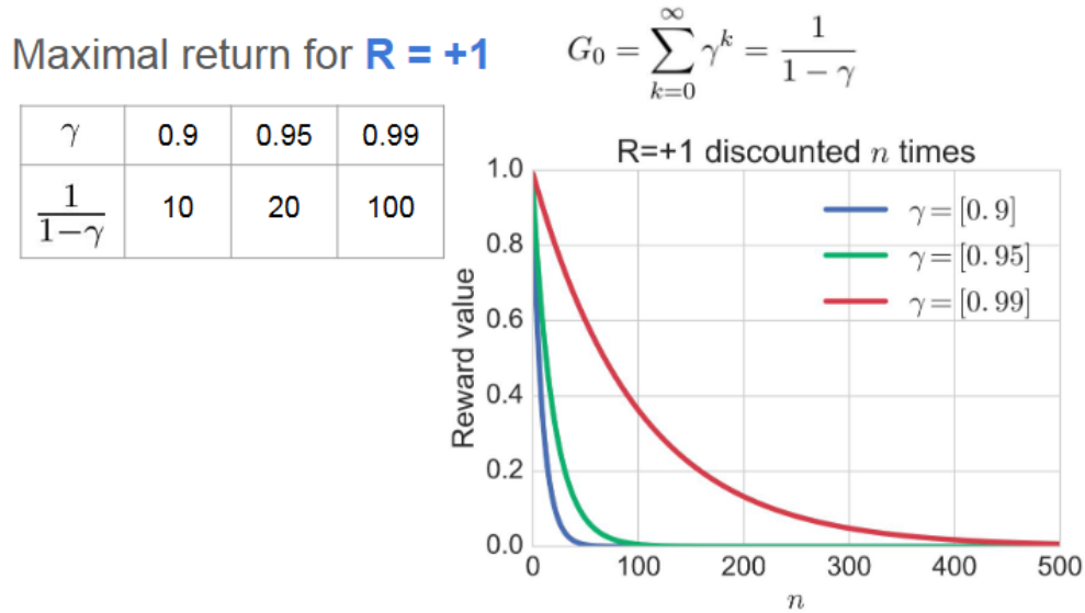
Figure 44: Discounting делает бесконечную сумму reward конечной.
