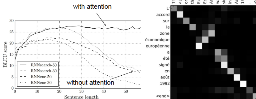
Figure 16: Преимущества attention: лучшее качество на длинных последовательностях и интерпретируемое выравнивание слов.
