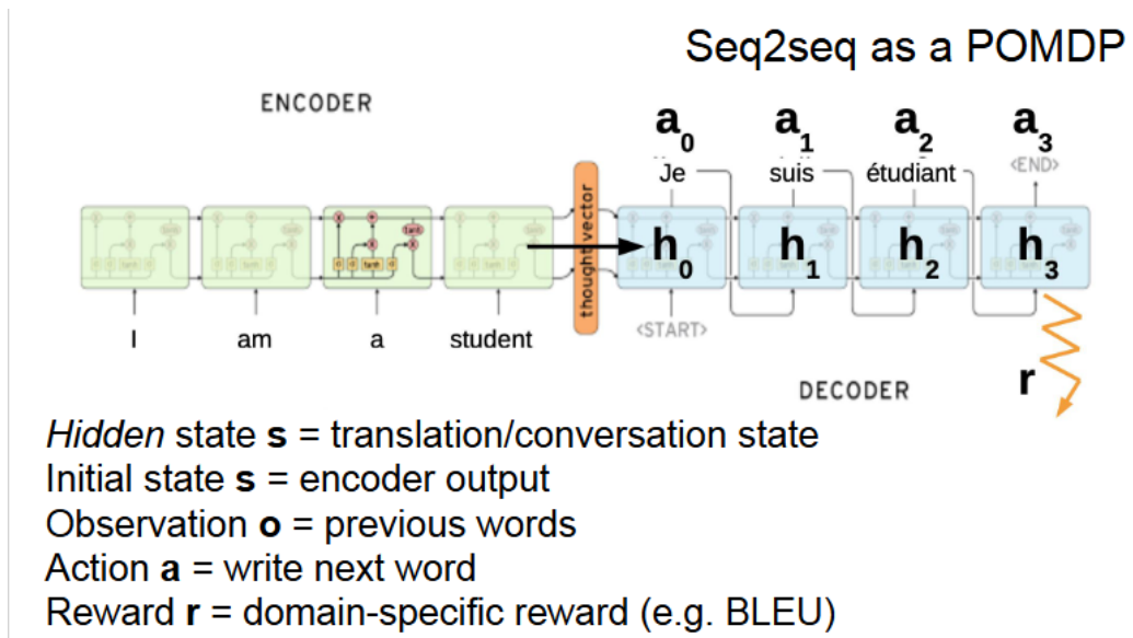
Figure 65: Seq2seq можно рассматривать как POMDP: decoder выбирает следующий токен как действие.
