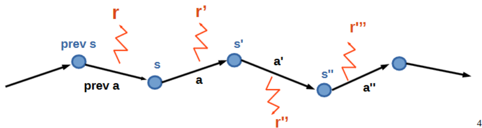
Figure 58: REINFORCE оценивает Q^\pi(s, a) через return G_t , посчитанный по sampled trajectory.
