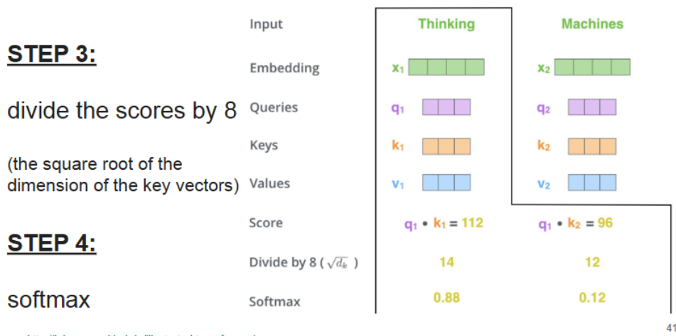
Figure 20: Scaled dot-product attention: scores масштабируются и нормируются softmax-ом.
