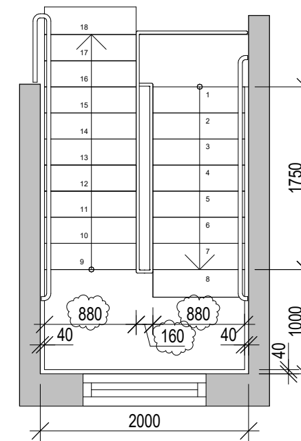
Översta Plan - förhöjd våning alt.1 1 : 50
