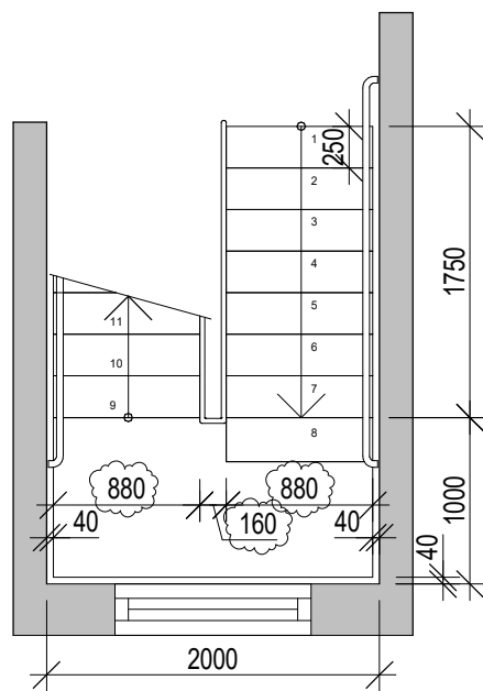
Första Plan 1 : 50
