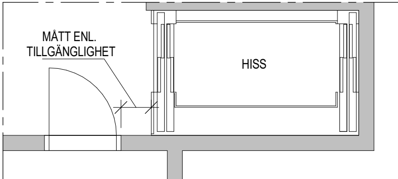
Alternativ 1 - normalplan 1 : 50
