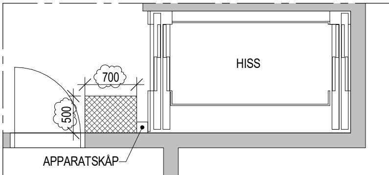
Alternativ 1 - översta planet 1 : 50
