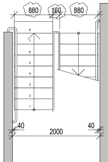
Första Plan 1 : 50
