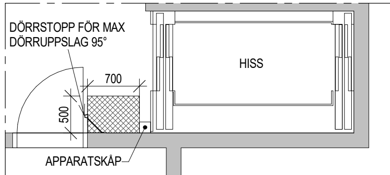
Alternativ 2 - översta planet 1 : 50
