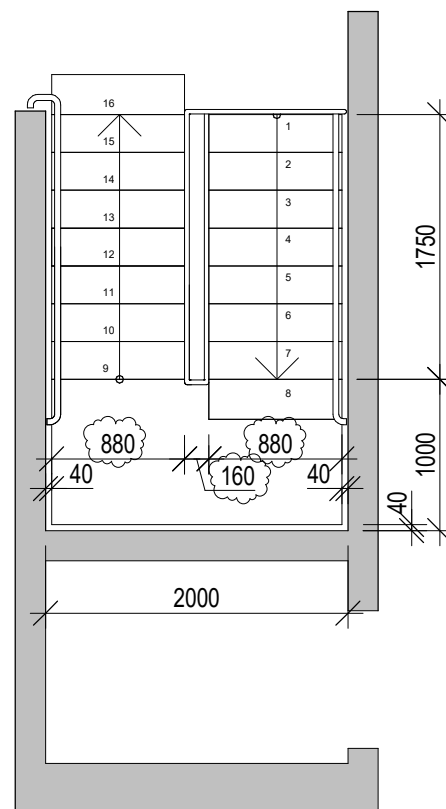
Översta Plan 1 : 50
