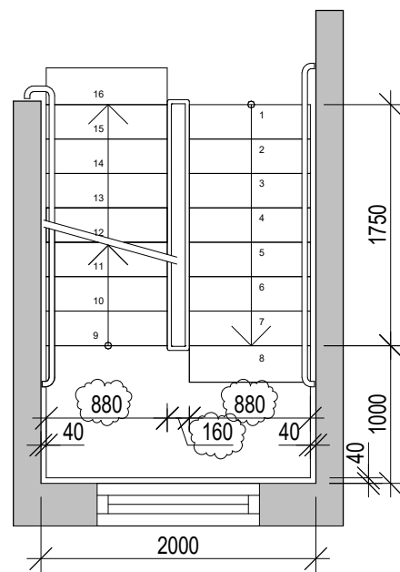
Normalplan 1 : 50
