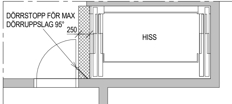
Alternativ 2 - normalplan 1 : 50
