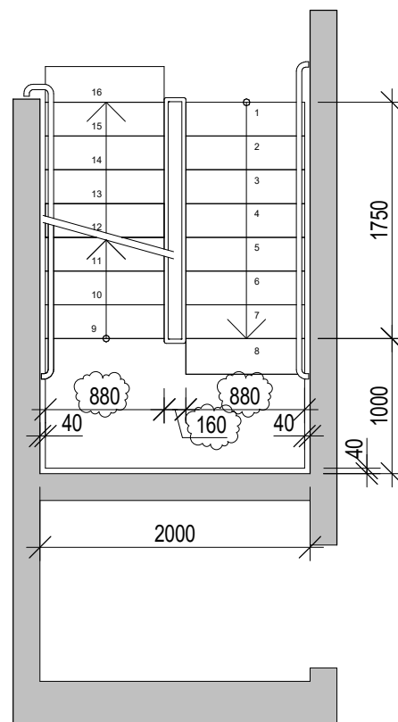
Normalplan 1 : 50
