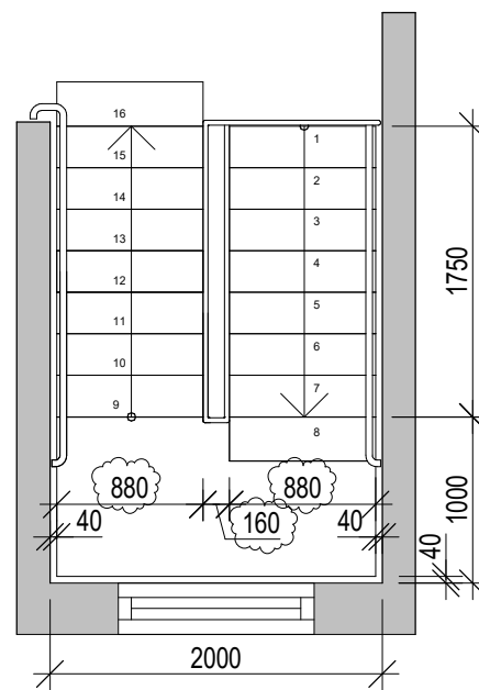
Översta Plan 1 : 50
