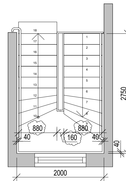
Översta Plan - förhöjd våning alt.2 1 : 50
