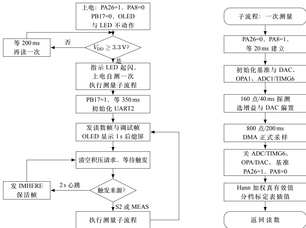
图 3 程序流程图
