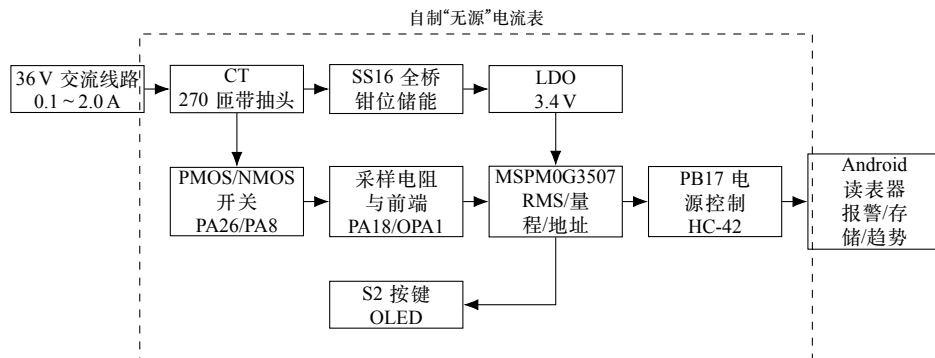
图 1 系统框图
