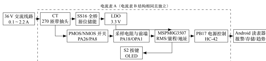
图 1 系统框图
