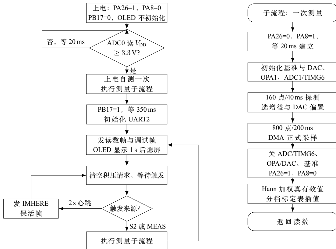
图 4 程序流程图
