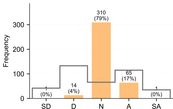
Qwen3-32B
