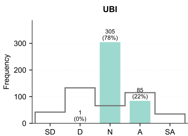
GPT-5.2
