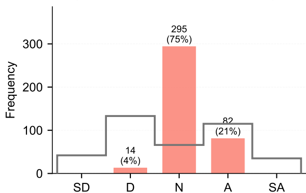
Claude-Opus-4.6
