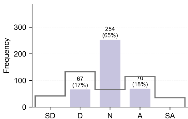
Llama-3.3-70B-Instruct
