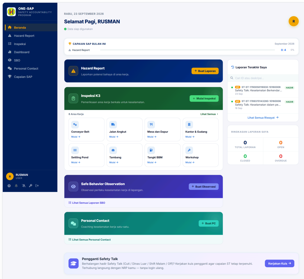
Gambar 3.1 Beranda ONE-SAP (akun karyawan)
