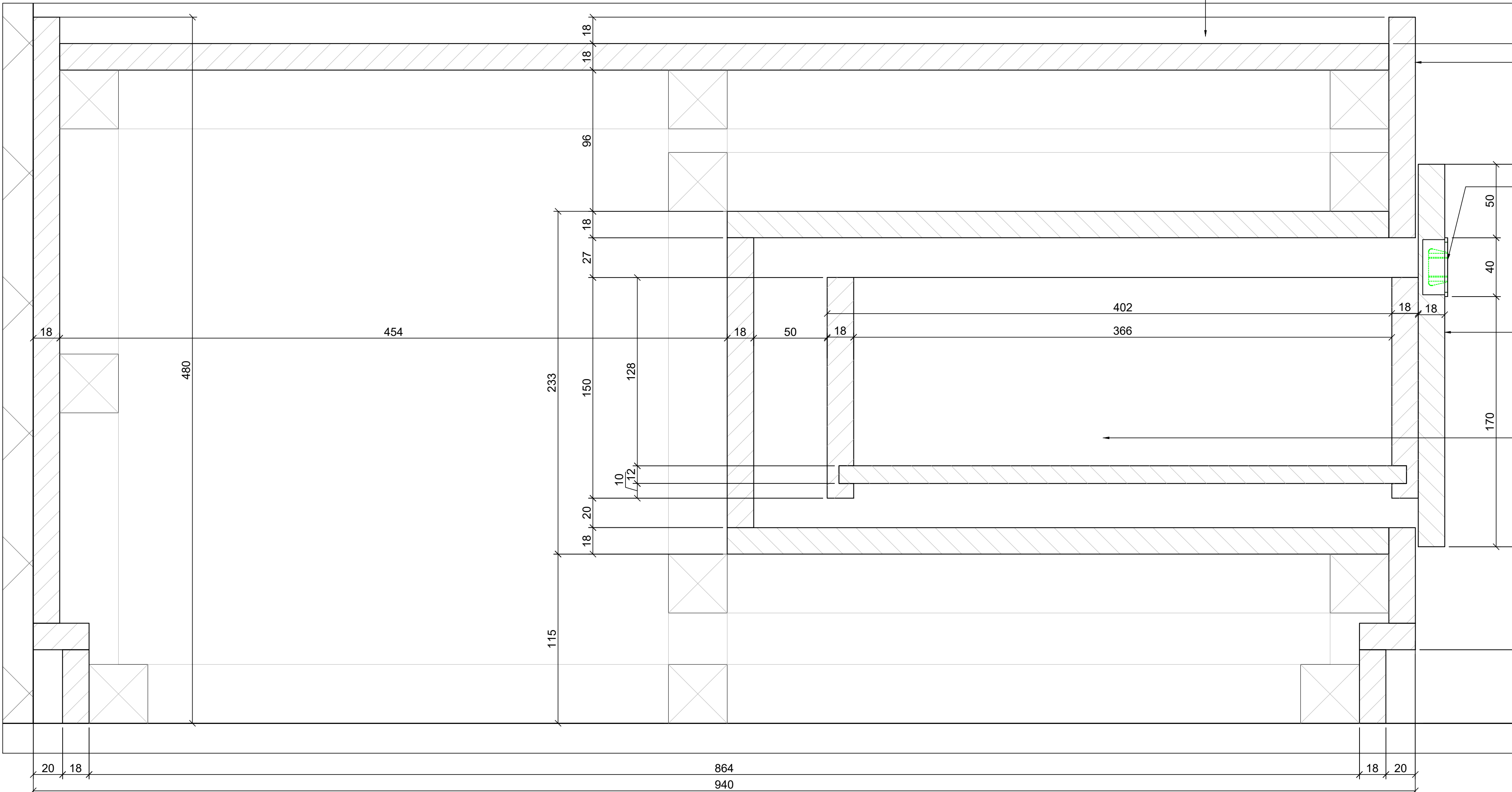
8 DETAIL Scale: 1:5
