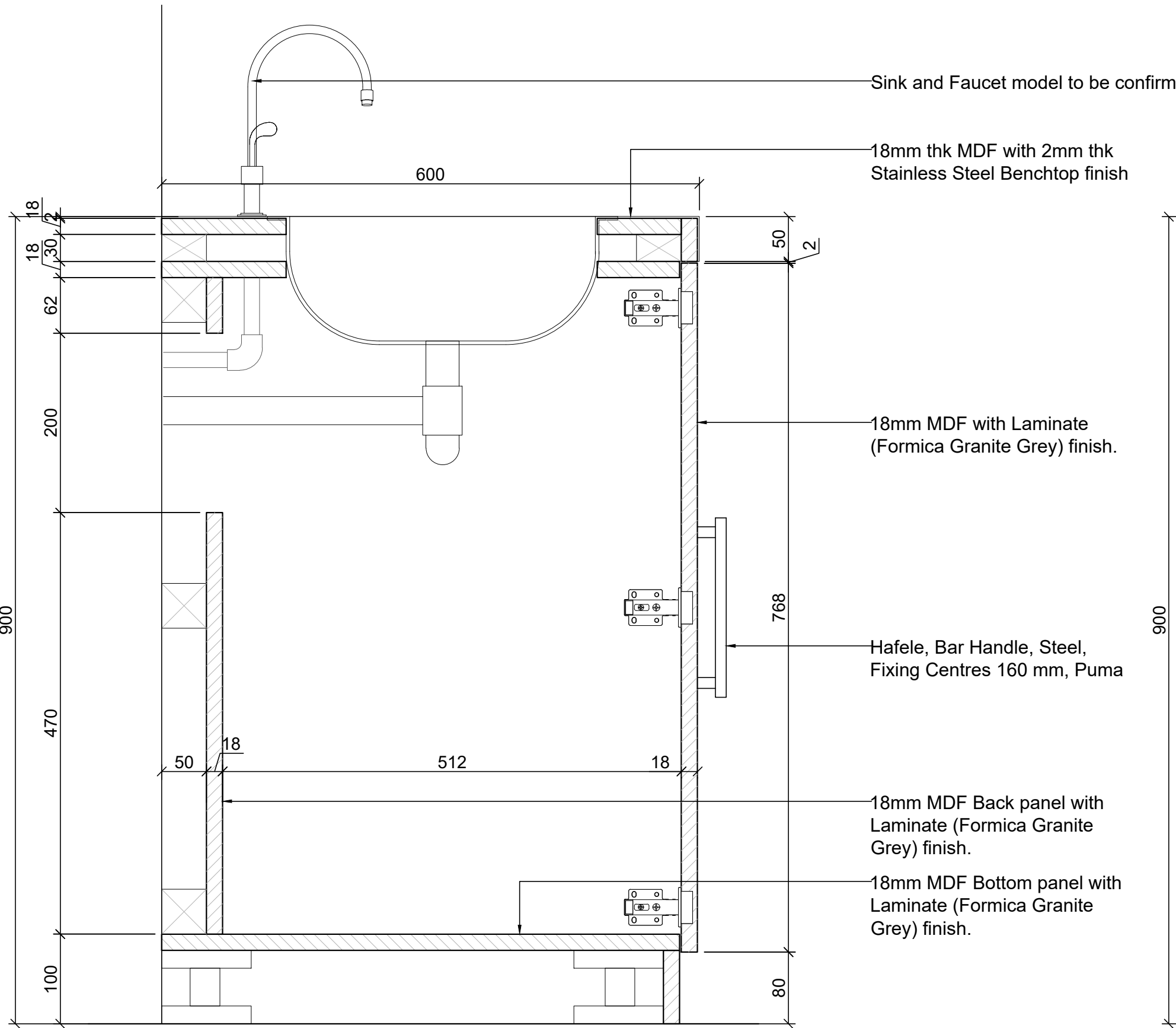
10 DETAIL Scale: 1:5
