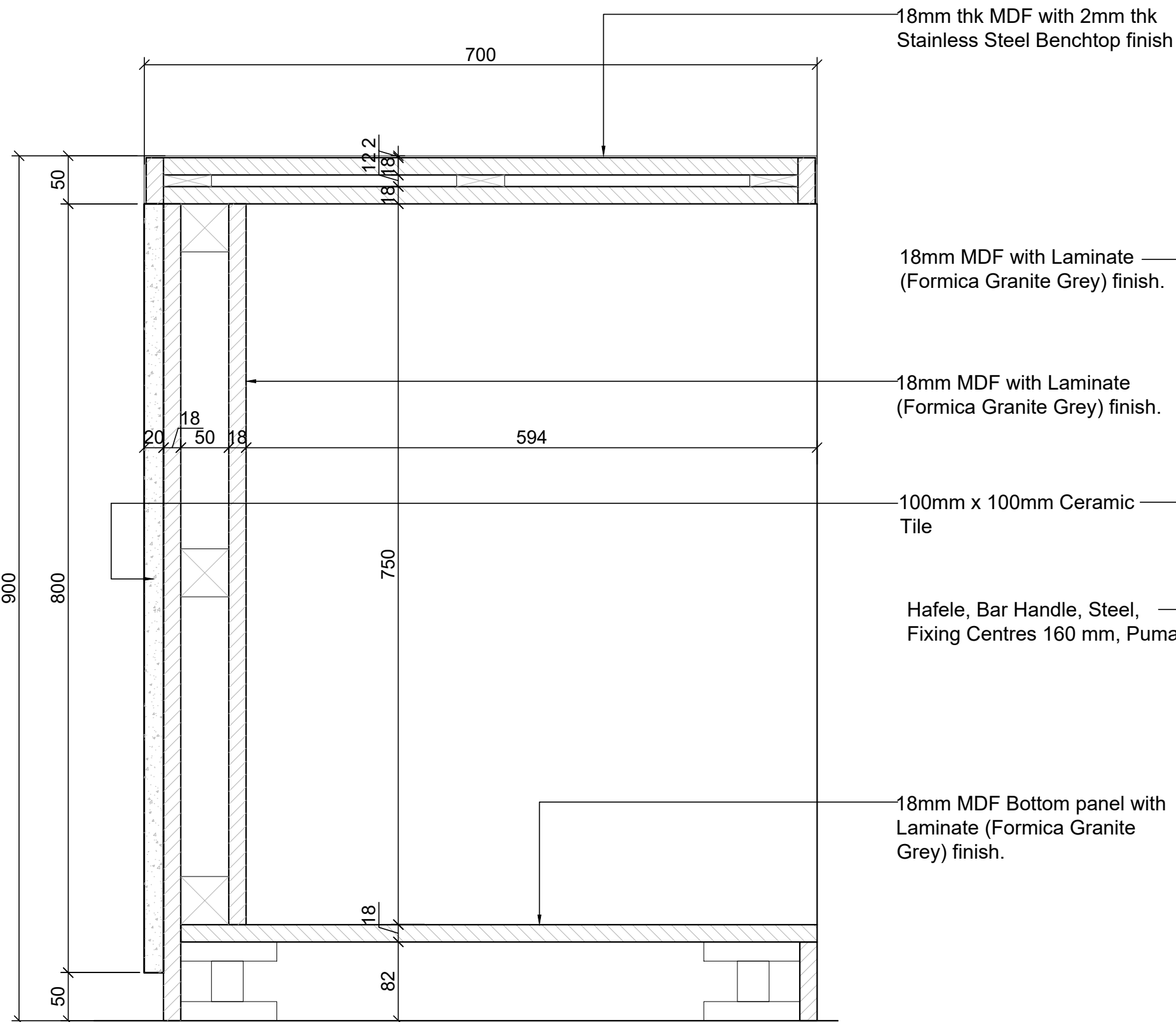
12 DETAIL Scale: 1:5
