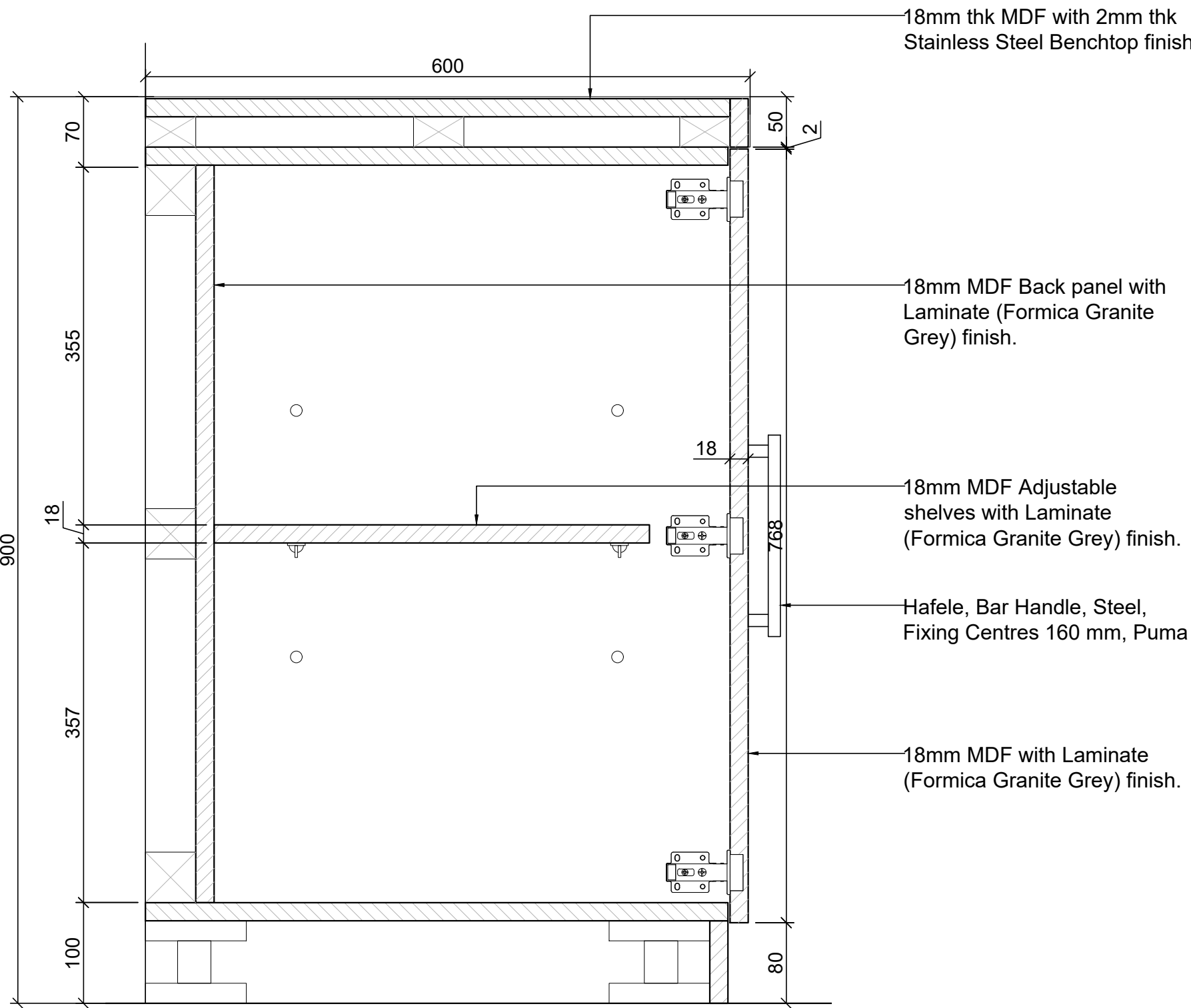
11 DETAIL Scale: 1:5
