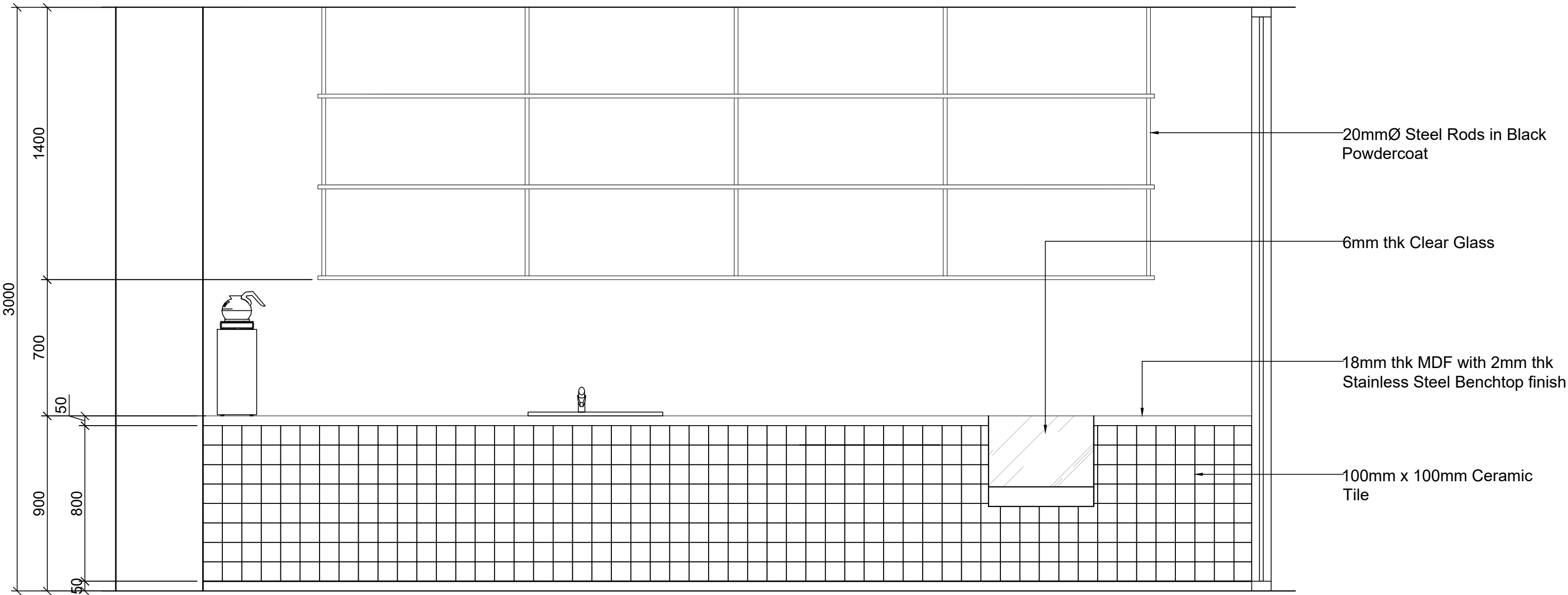
5 ELEVATION
