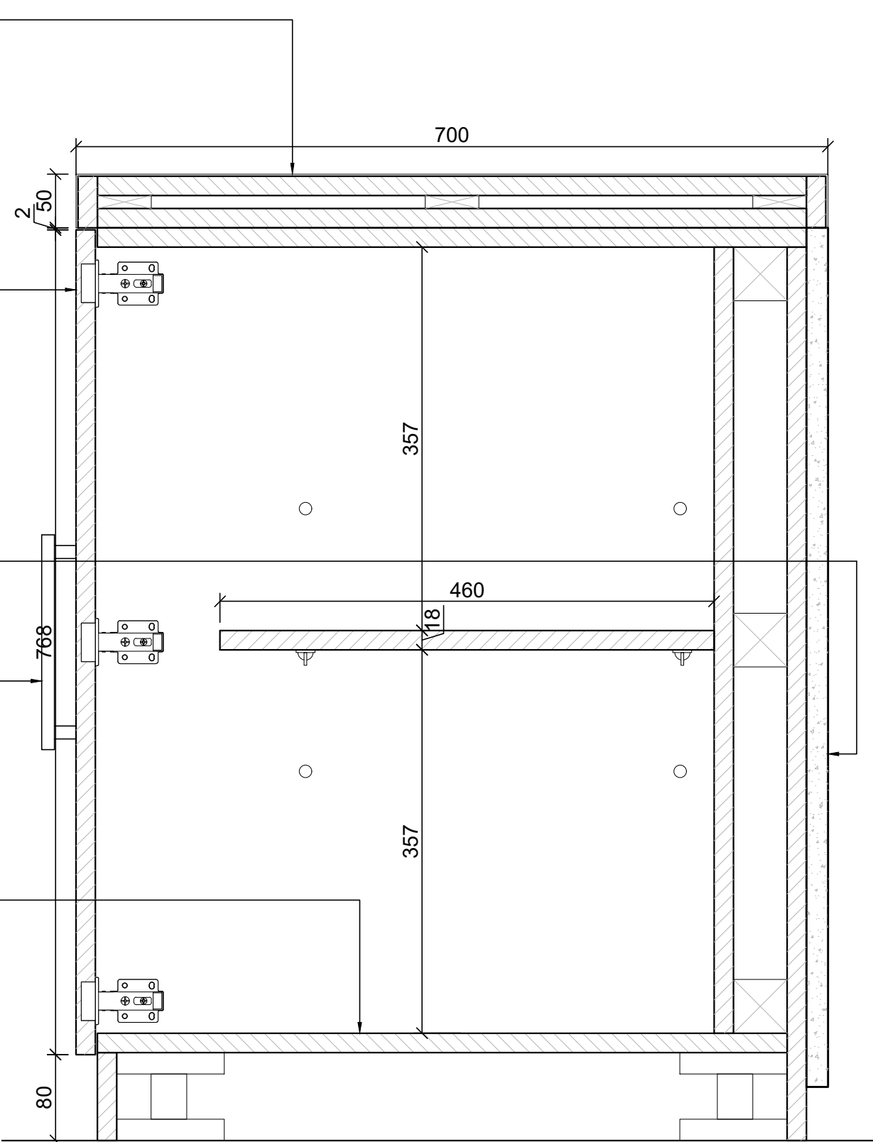
13 DETAIL Scale: 1:5
