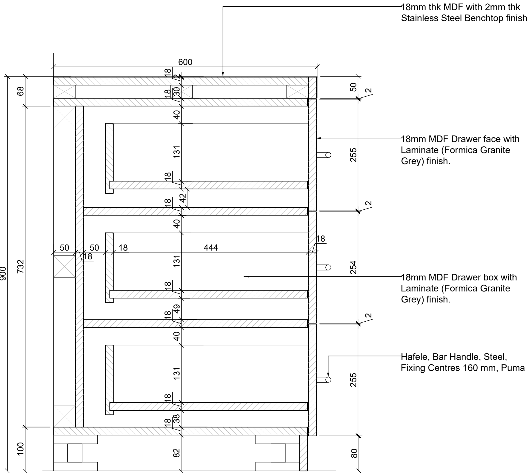
09 DETAIL Scale: 1:5
