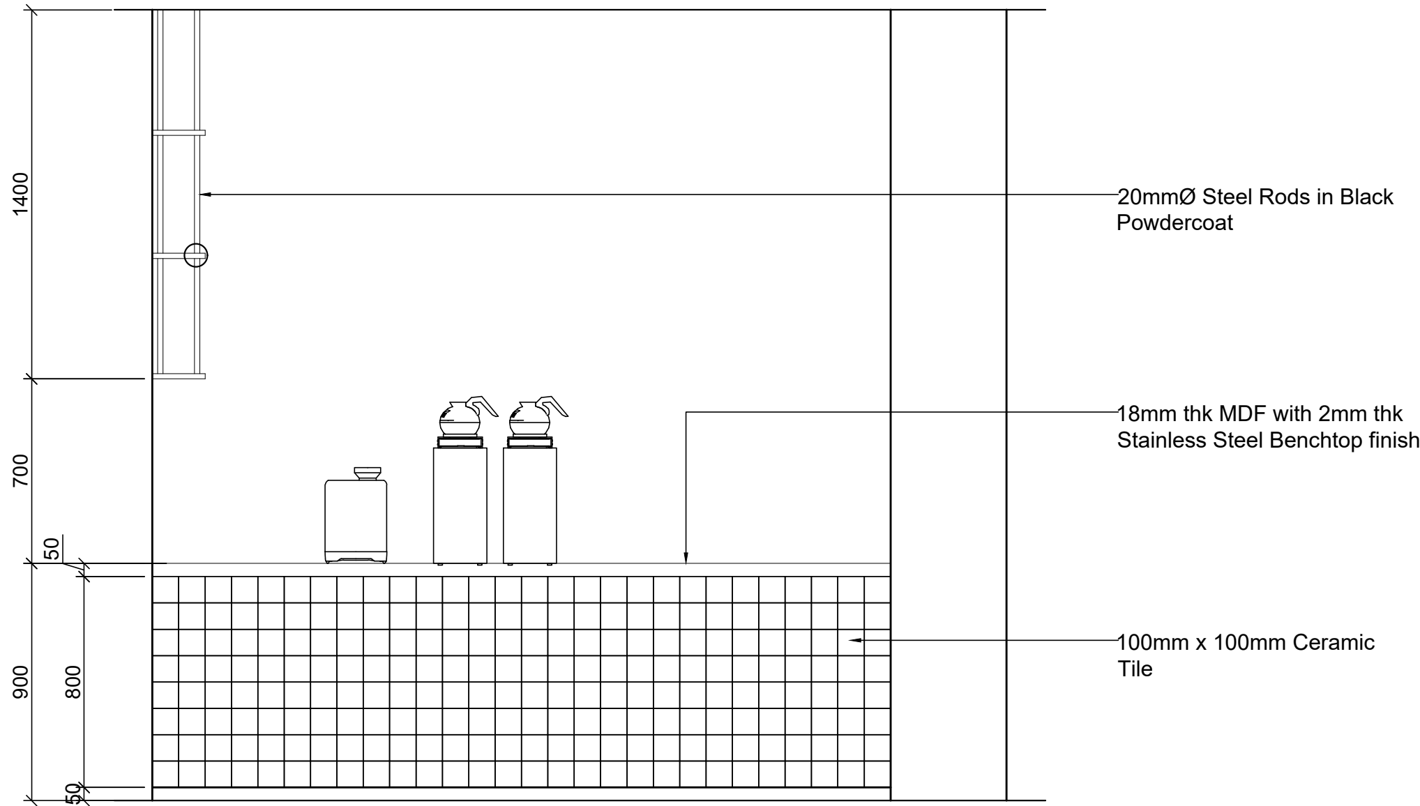
6 ELEVATION
