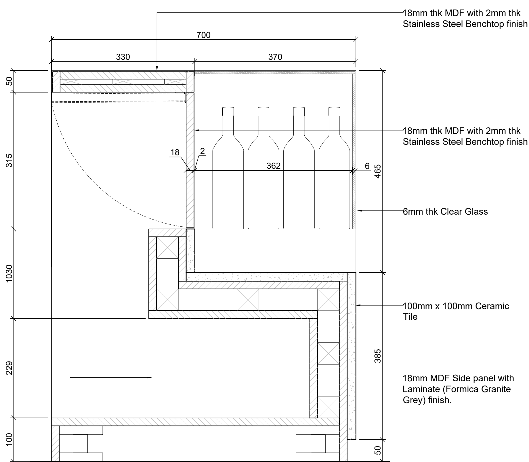
14 DETAIL Scale: 1:5
