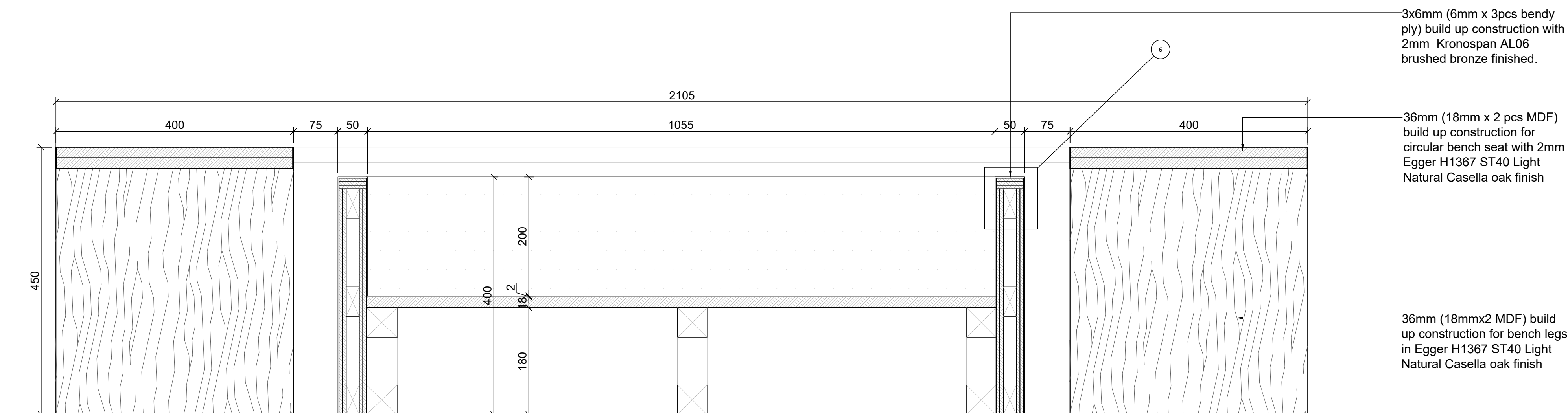
4 SECTION Scale: 1:5
