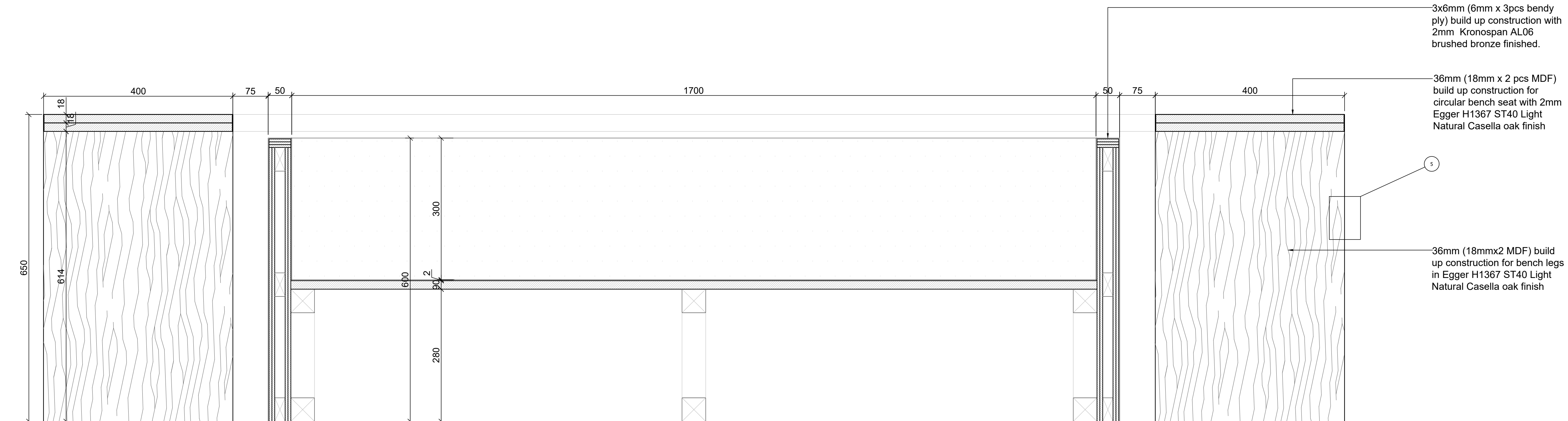
3 SECTION _____ Scale: 1:5
