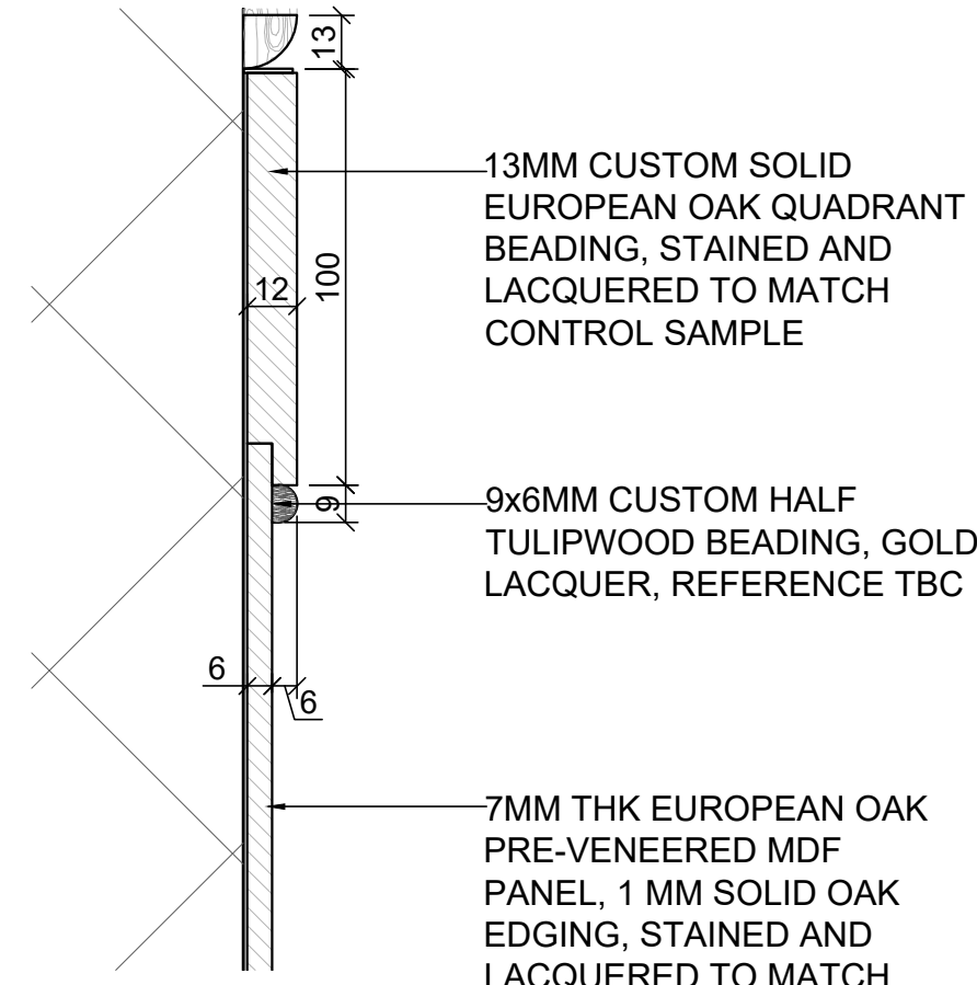
12 DETAILS Scale: 1:2
