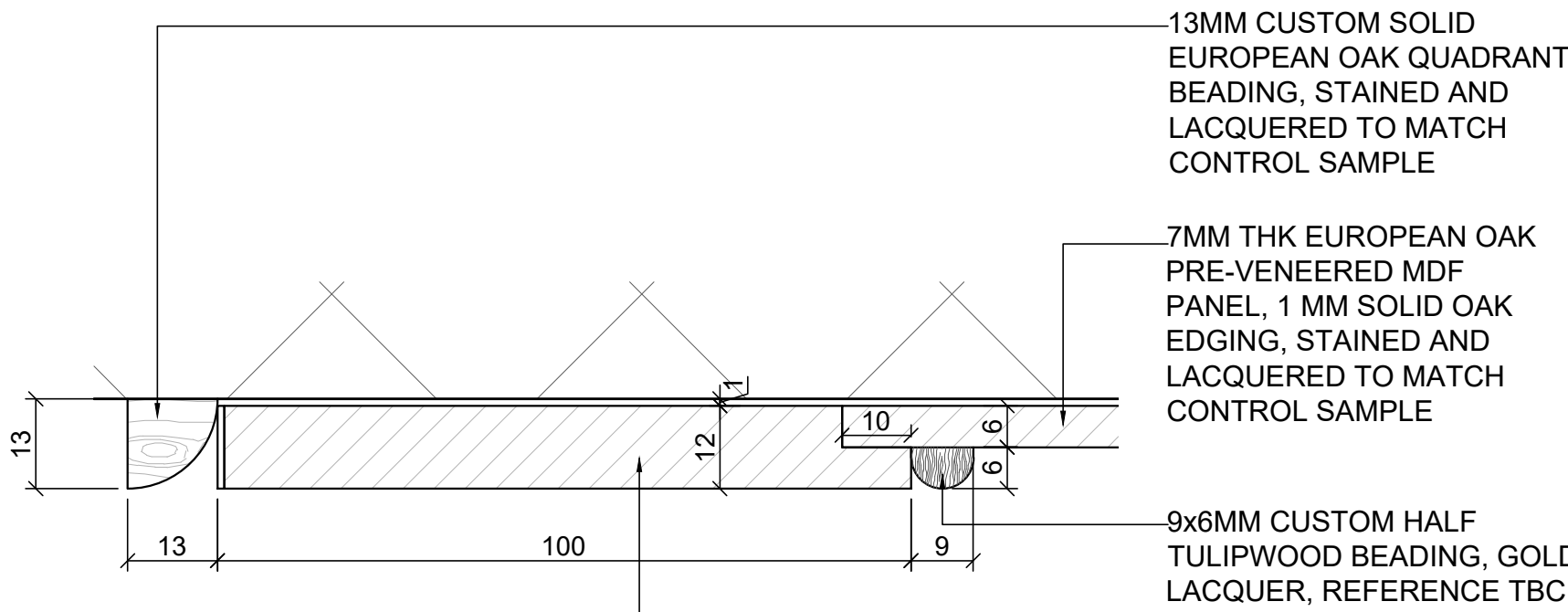
11 DETAILS Scale: 1:1
