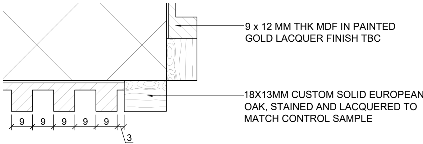
9 DETAILS Scale: 1:1
