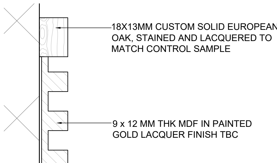
10 DETAILS Scale: 1:1
