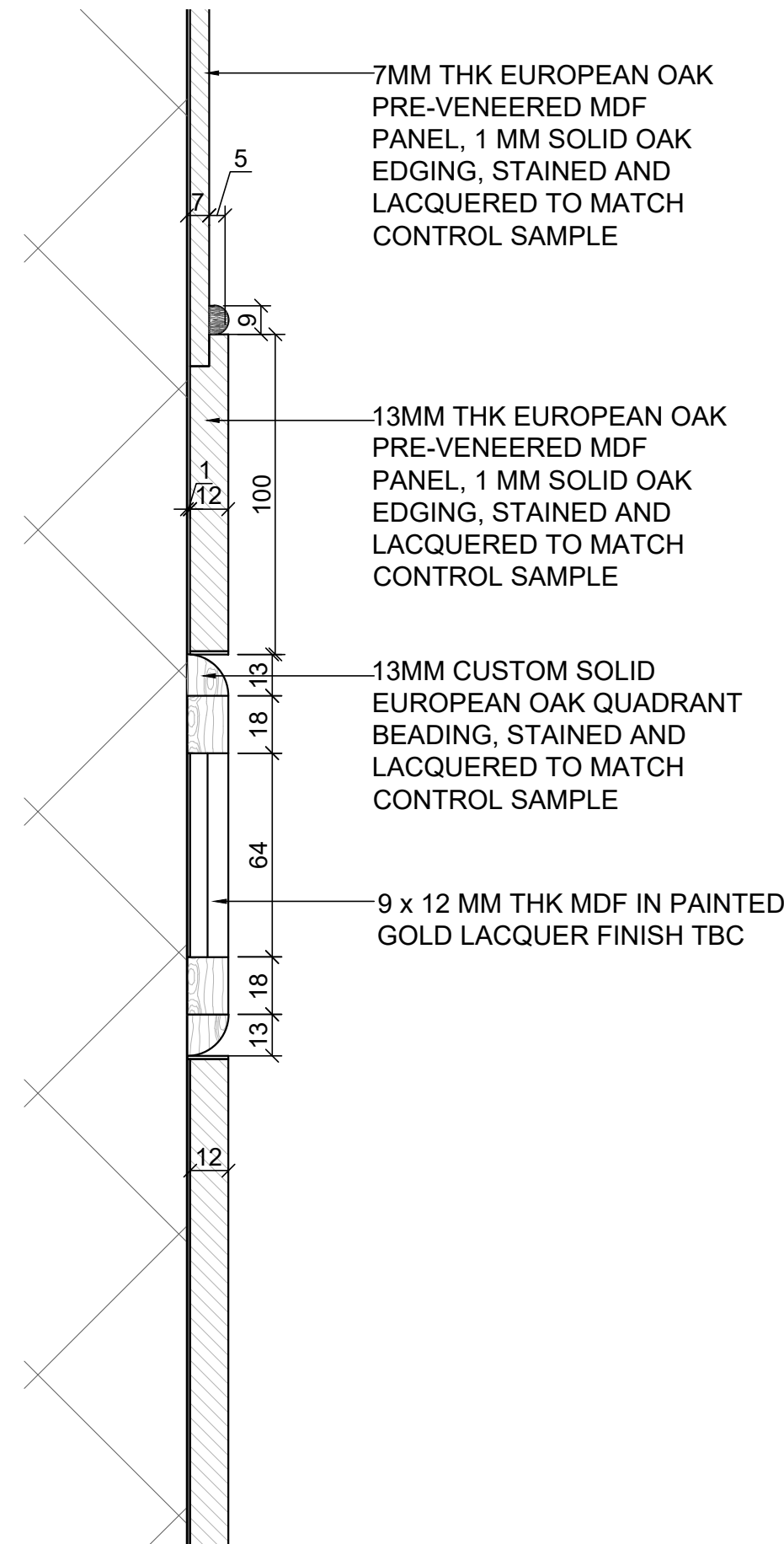
13 DETAILS Scale: 1:2
