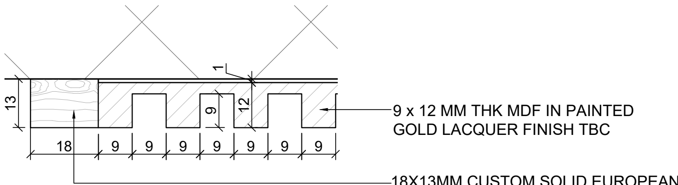
8 DETAILS Scale: 1:1
