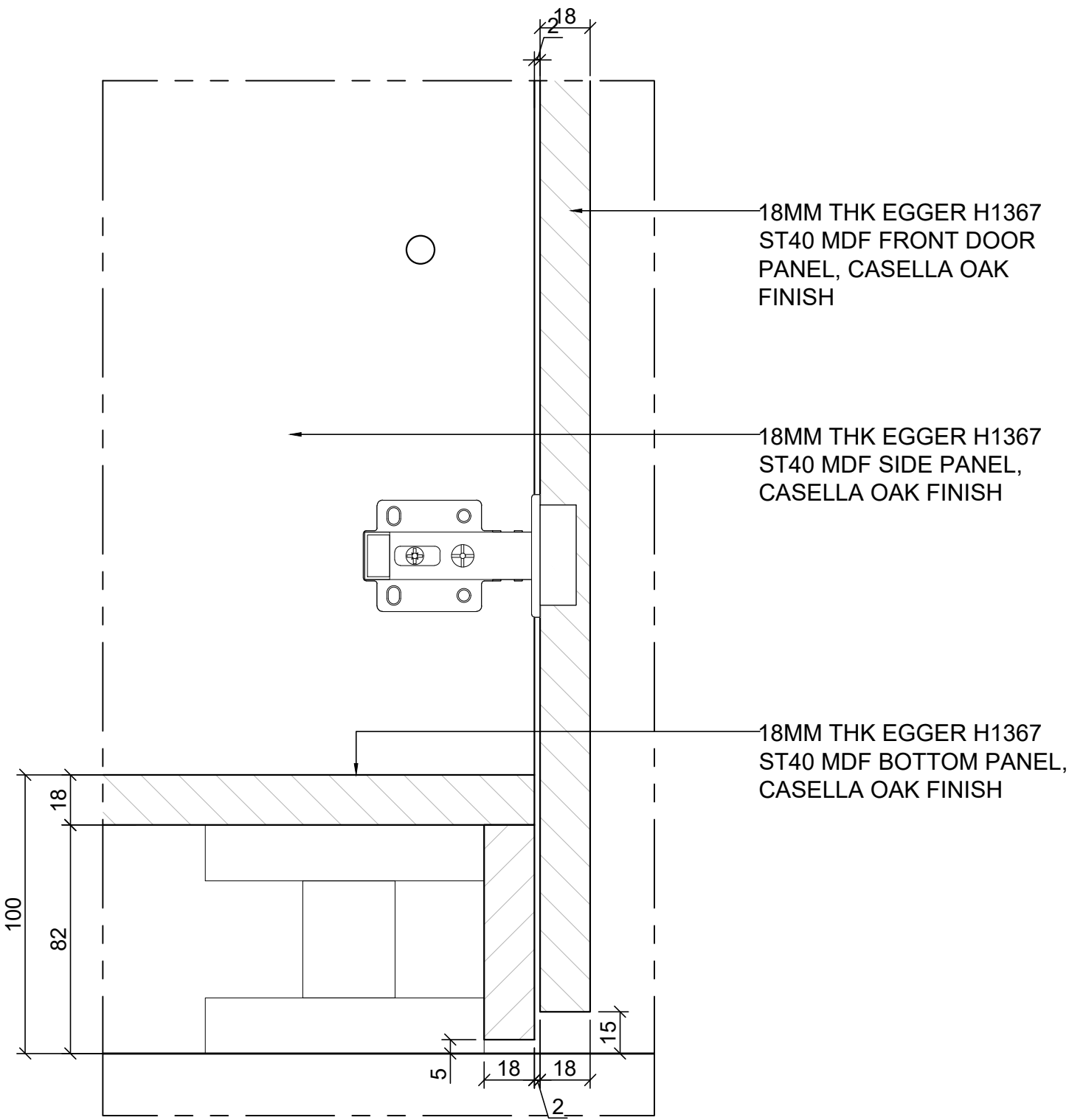
7 DETAIL Scale: 1:2
