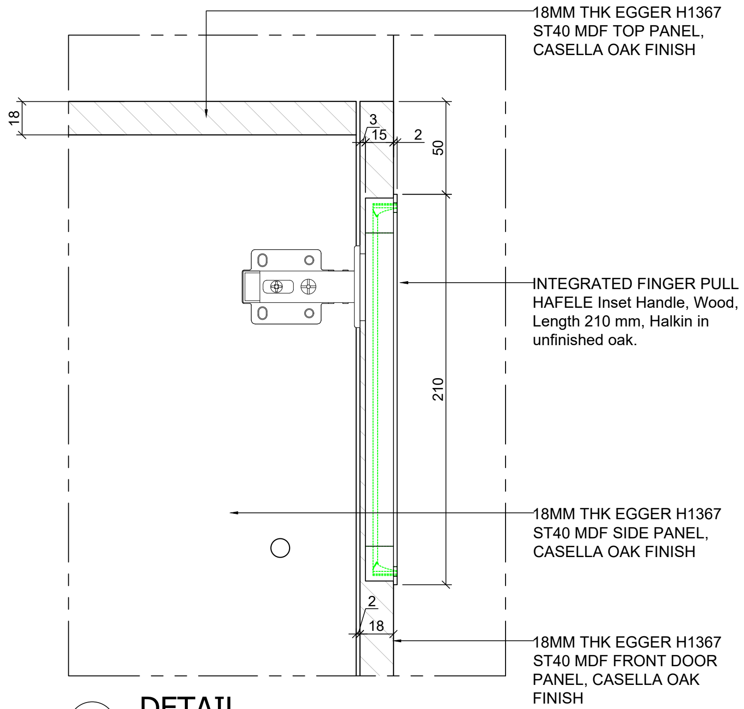
6 DETAIL Scale: 1:2
