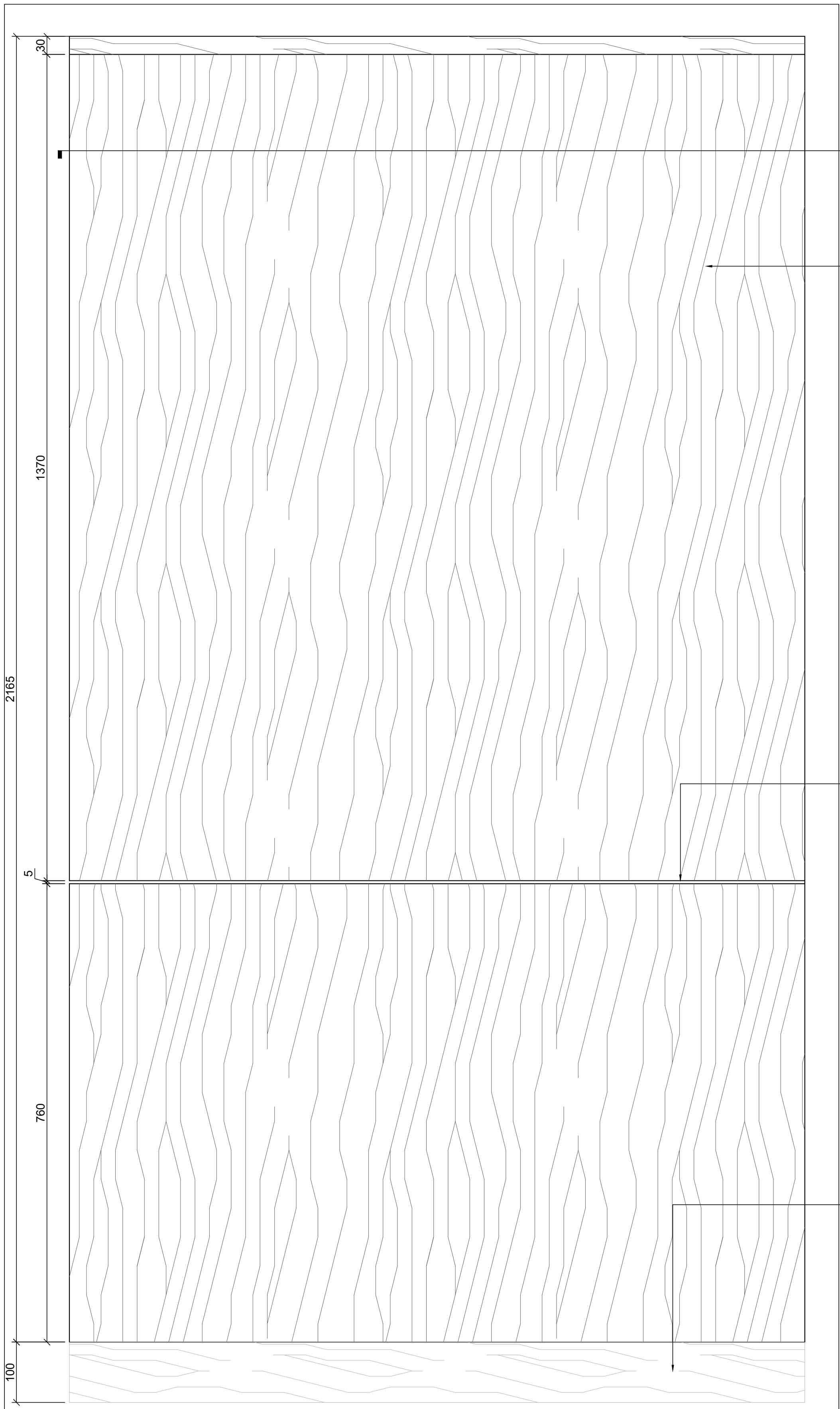
2 ELEVATION Scale: 1:5
