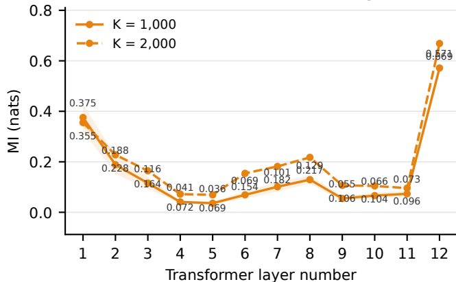
MusicBERT SOD: Tempo
