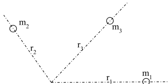
Figure 7: Distancias de varias masas al punto donde se calcula el potencial.
