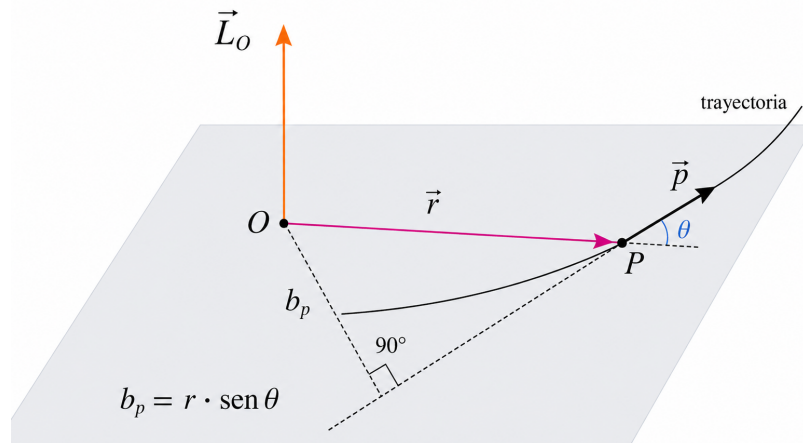
Figure 3: Vectores posición, cantidad de movimiento y momento angular.
