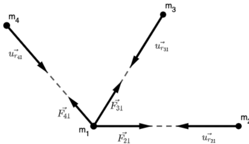
Figure 5: Superposición de las fuerzas gravitatorias ejercidas sobre la masa 1.
