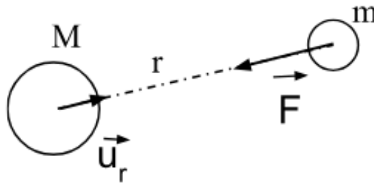
Figure 4: Interacción gravitatoria entre dos masas.
