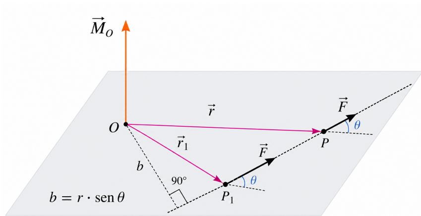
Figure 1: Vectores posición, fuerza y momento respecto de un punto.
