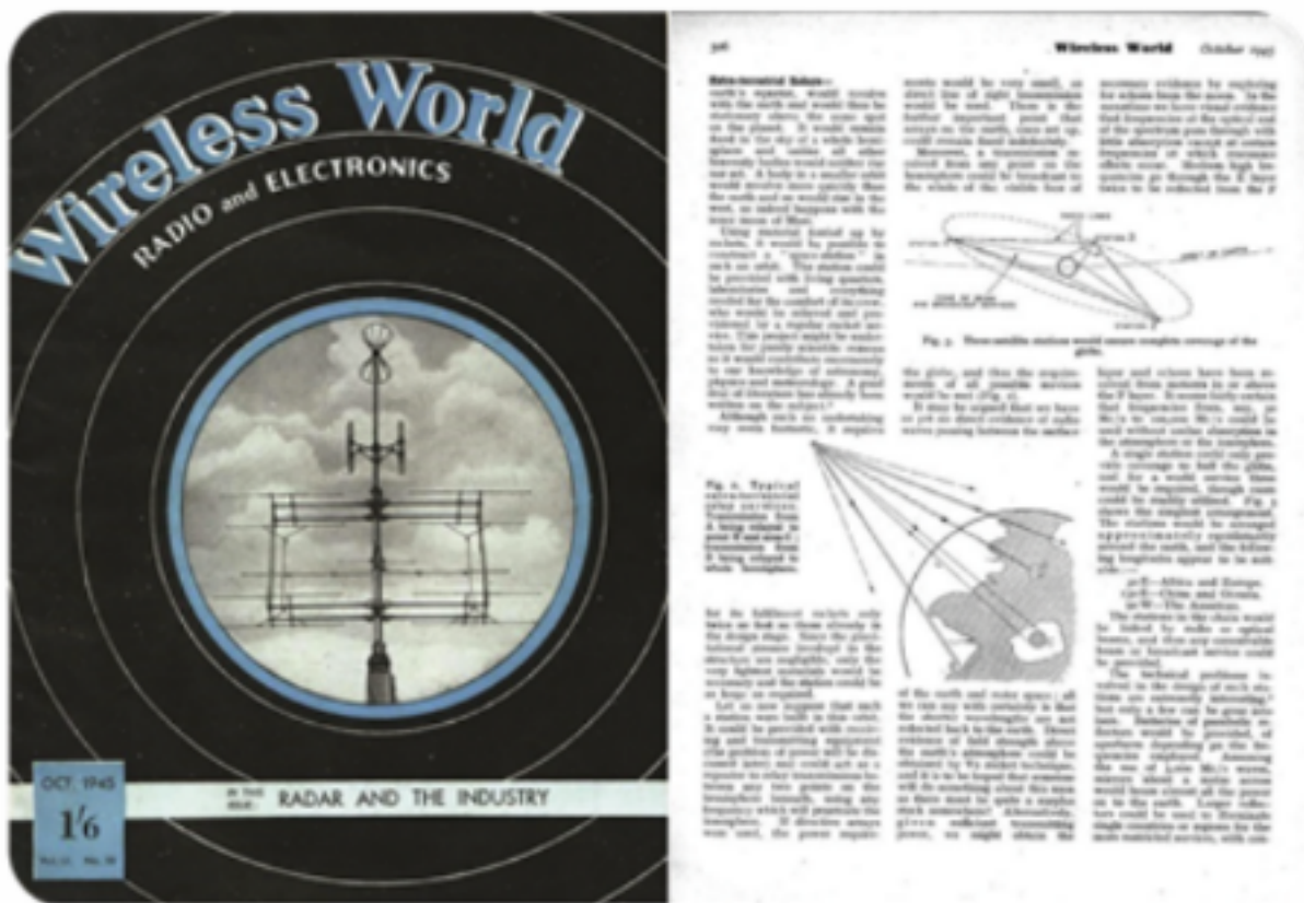
Figure 16: Artículo de Arthur C. Clarke sobre órbitas geoestacionarias
