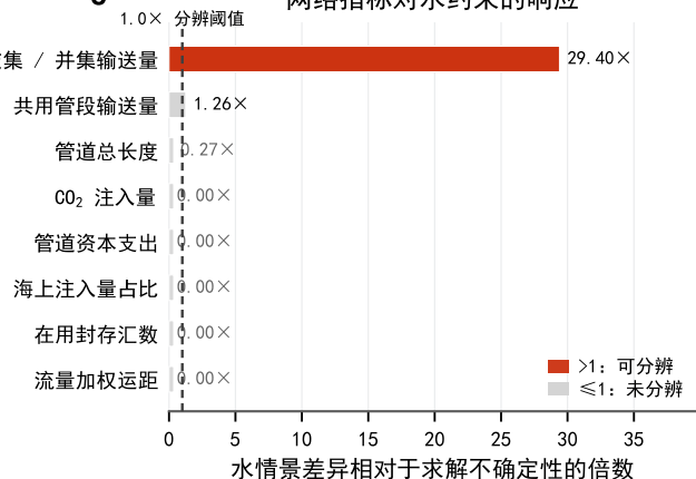
网络指标对水约束的响应
