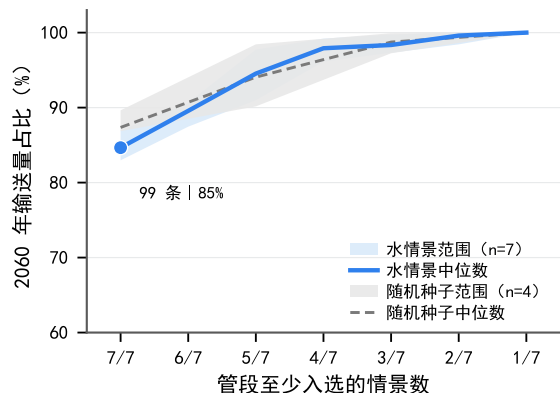
核心管段承担的输送量
