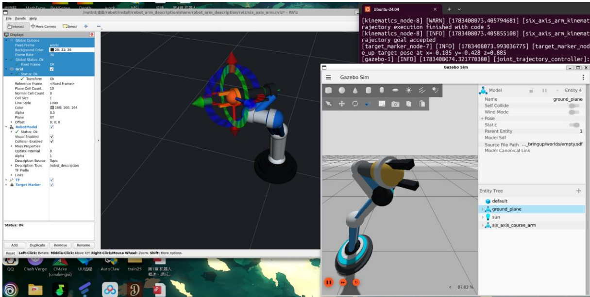
图 6 RViz 交互控制、Gazebo 仿真与终端日志的同步运行截图
