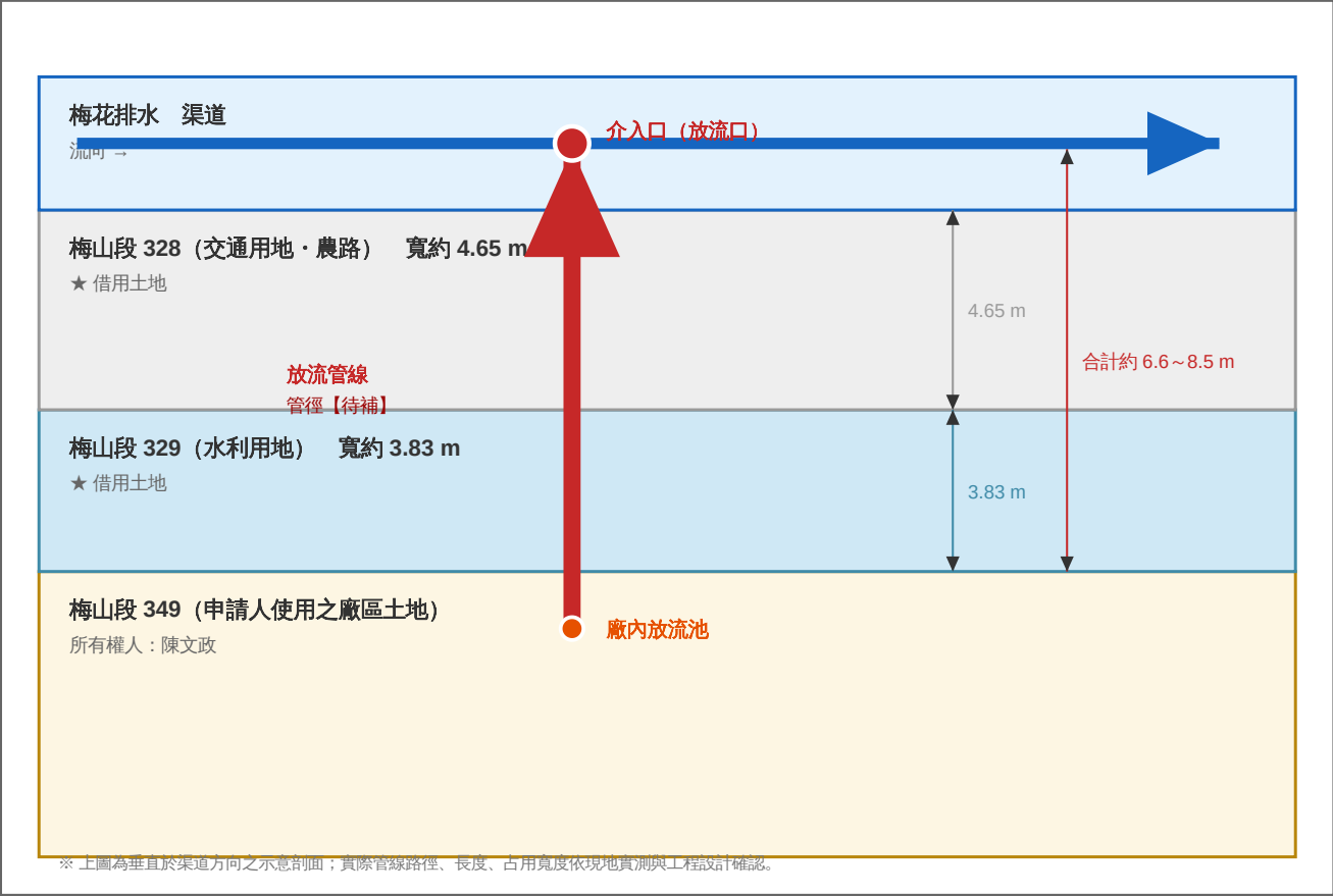
圖四 借用他人土地 管線位置圖說
