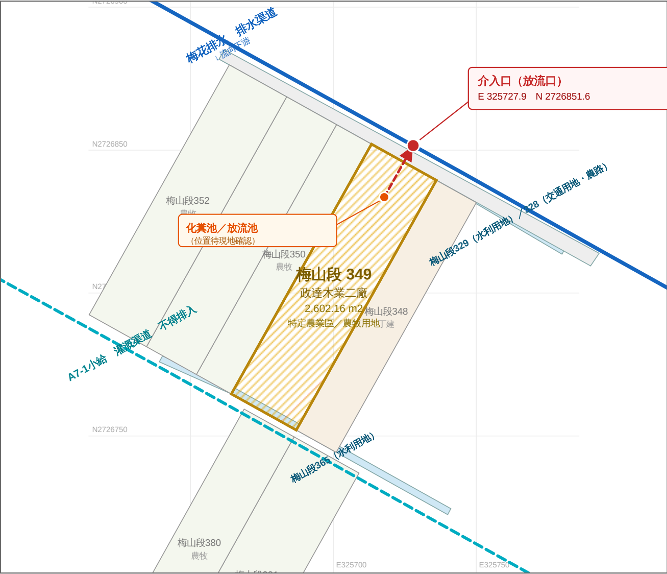
圖二 介入點位置圖（平面圖）
