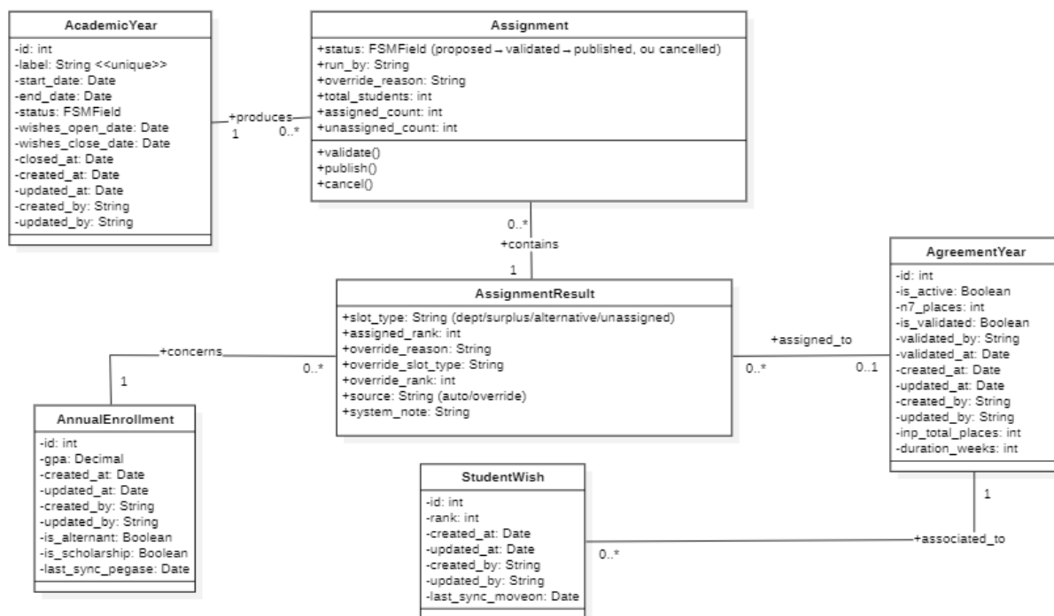
FIGURE 5.9 – Diagramme de classes : Sprint 3
