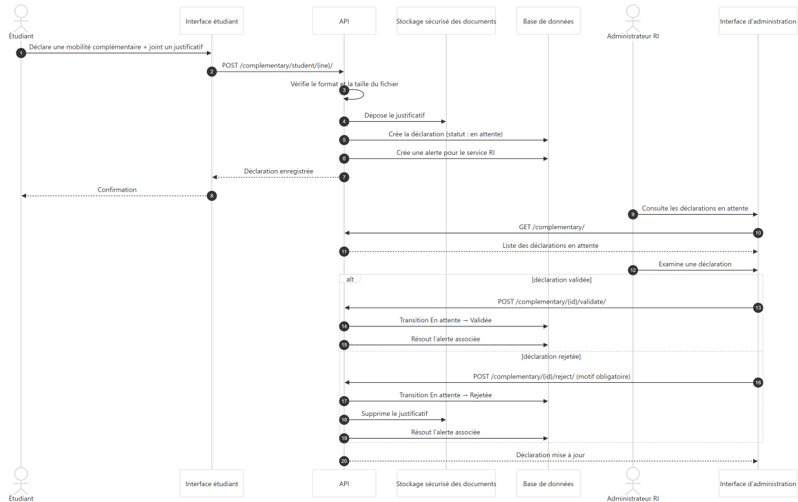
FIGURE 5.18 – Déclaration et traitement d'une mobilité complémentaire
